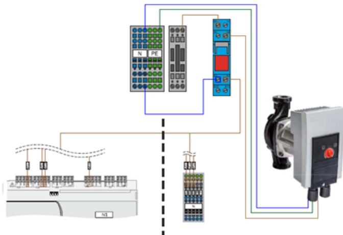
232 Abbildung: Anschlussschema Koppelrelais
