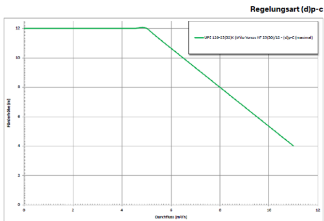
255 Abbildung: Kennlinien UPE 120-25(32)K
