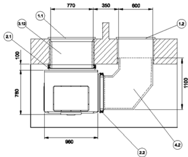
44 Abbildung: Draufsicht - LI 12TU und LI 16I-TUR (Wand-Aufstellung mit Luftkanal auf der Ausblasseite)
