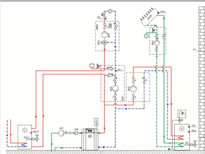
215 Abbildung: Einbindungsschema für den monoenergetischen Wärmepumpenbetrieb, einem Heizkreis, Reihen-Pufferspeicher mit externer Heizungsunterstützung und Warmwasserbereitung (Die Hydraulik ist nur für Sole- bzw. Wasser- bzw. Wasser/Wasser-Wärmepumpen geeignet)
