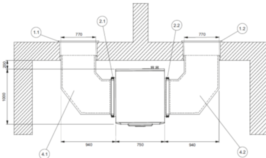
53 Abbildung: Draufsicht - LI 1422C und LI 1826C (Wand-Aufstellung mit Luftkanal auf der Ansaug- und Ausblasseite)
