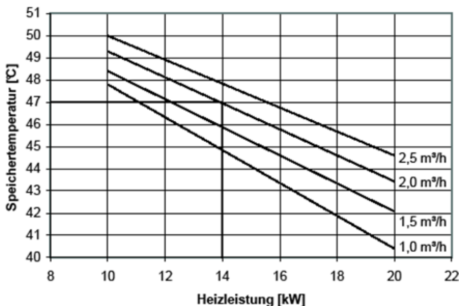
108 Abbildung: Auslegung eines Warmwasserspeichers am Beispiel WWSP 442
