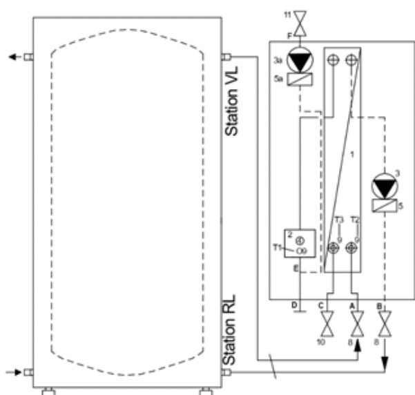
117 Abbildung: Funktionsdarstellung Frischwasserstation
