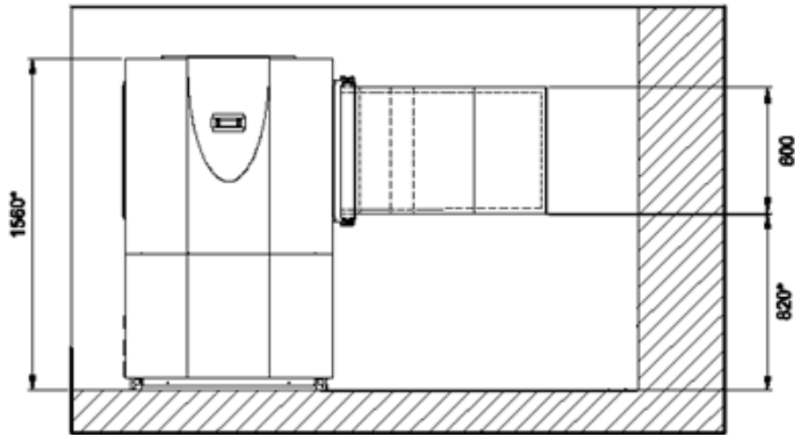
45 Abbildung: Frontansicht - LI 12TU und LI 16I-TUR (Wand-Aufstellung mit Luftkanal auf der Ausblasseite) LIK 12TU - Eck-Aufstellung
