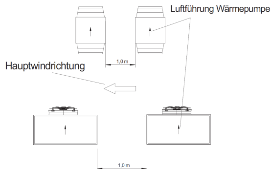
18 Abbildung: Parallelschaltung von Wärmepumpen
