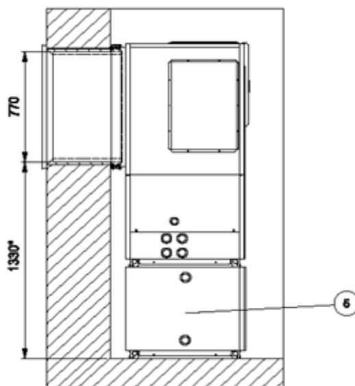
33 Abbildung: Seitenansicht - LI 12TU und LI 16I-TUR (Wand-Aufstellung - Luftkanal Ausblasseite)
