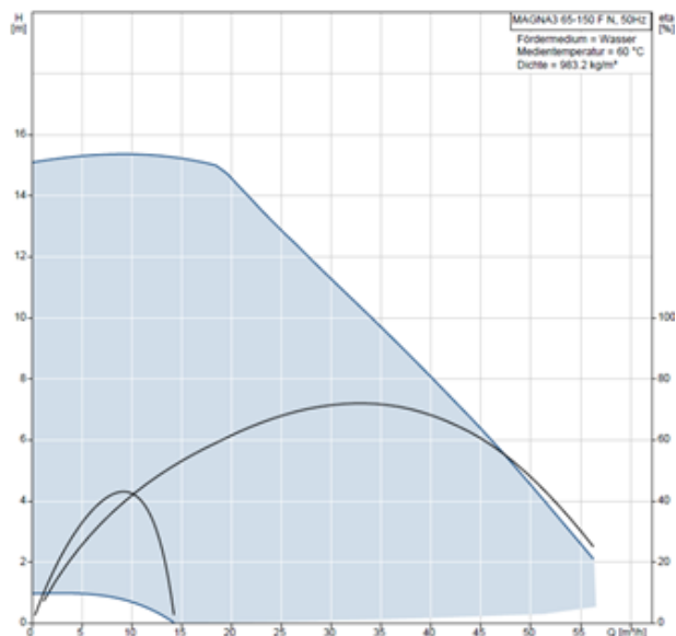
317 Abbildung: Förderhöhe Magna3 65-150F
