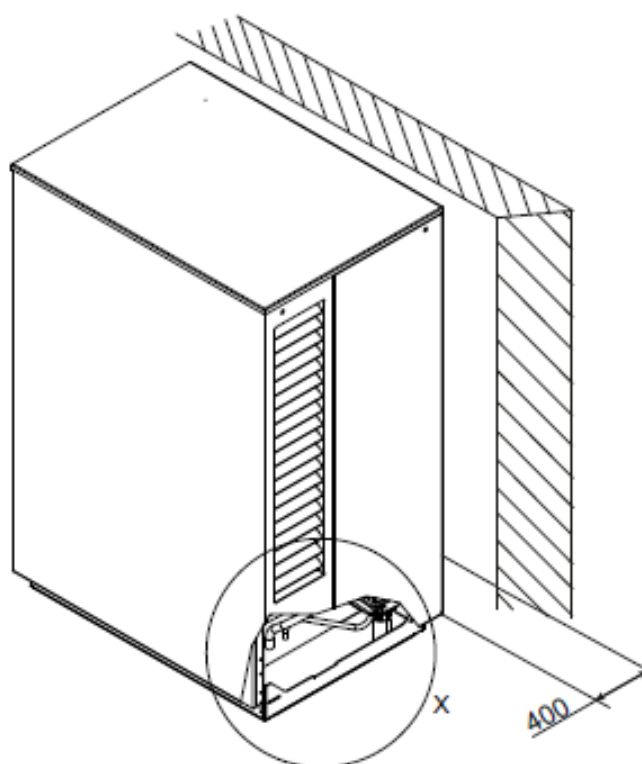
59 Abbildung: Aufstellung Außeneinheit M Flex und System M Comfort
