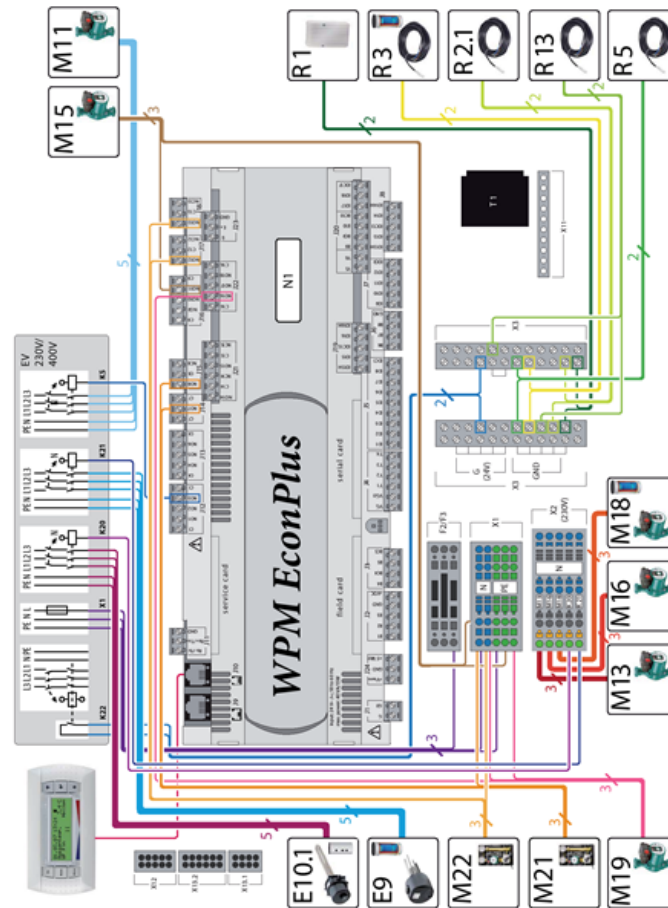
219 Abbildung: Wärmepumpenmanager WPM EconPlus bei bivalenten Anlagen mit einem Heizkreis und konstant- oder gleitend geregeltem Heizkessel
