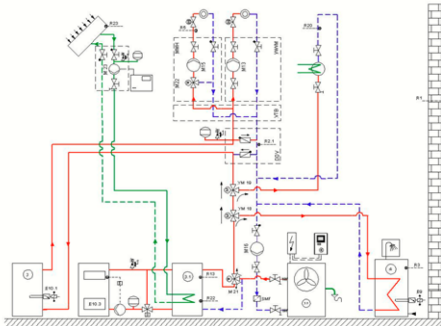
218 Abbildung: Einbindungsschema für den monoenergetischen Wärmepumpenbetrieb mit zwei Heizkreisen, Warmwasser- und Schwimmbaderwärmung
