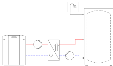
104 Abbildung: Ladespeicher mit externem Wärmetauscher
