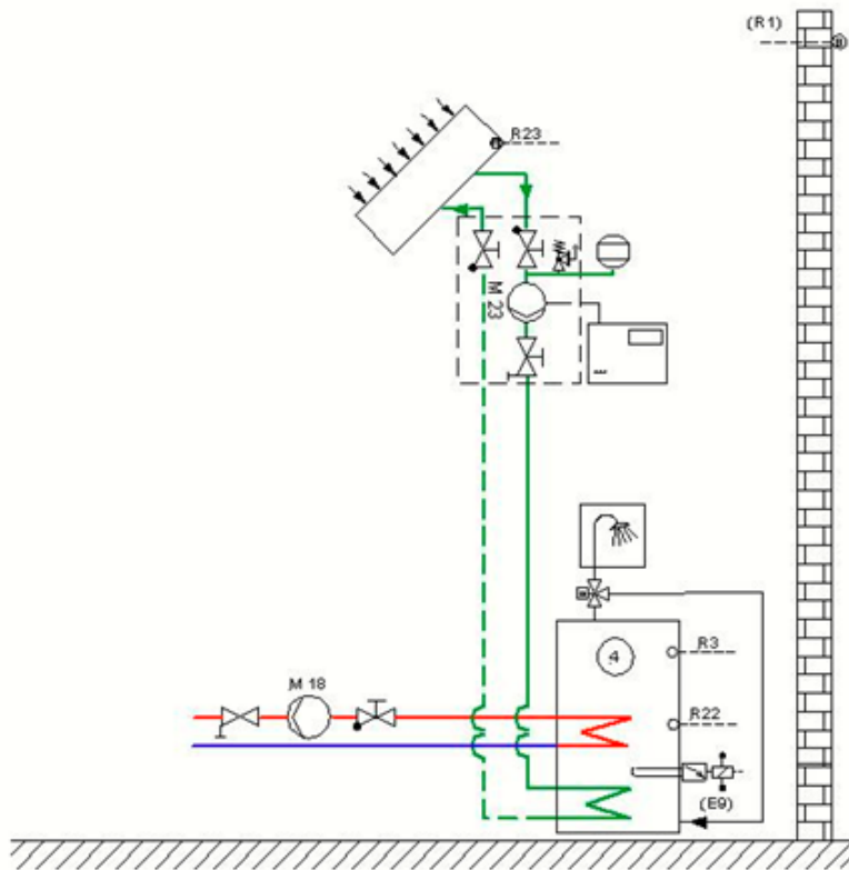
214 Abbildung: Einbindungsschema (ohne Sicherheitsarmaturen) der Wärmepumpe mit solarer Warmwasser-Unterstützung in Verbindung mit einer Solarstation.
