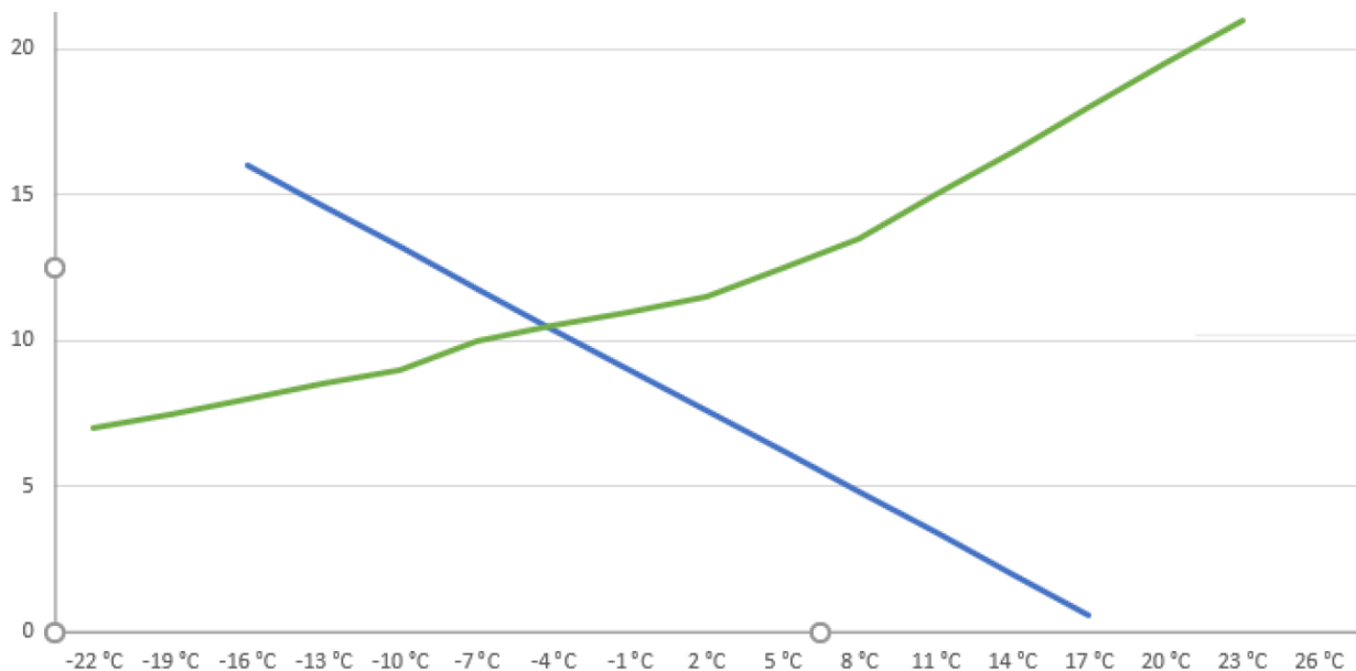
2 Abbildung: Heizleistungskurve Wärmepumpe mit einer Leistungsstufe (Fixed-Speed)
