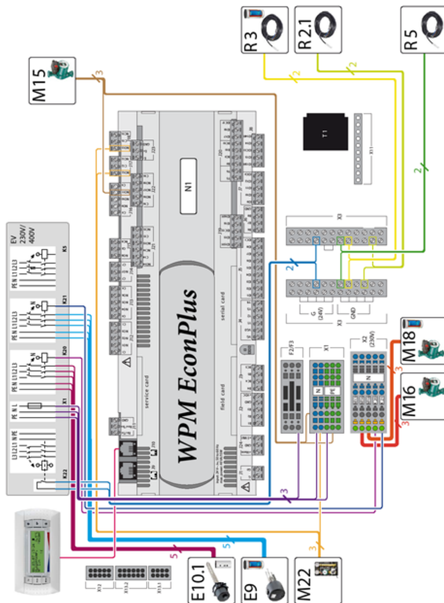
216 Abbildung: Wärmepumpenmanager WPM EconPlus bei bivalenten Anlagen mit einem Heizkreis und konstant- oder gleitend geregeltm Heizkessel
