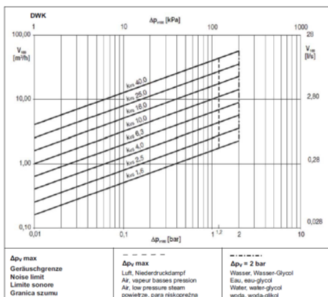
153 Abbildung: Druckverlustdiagramm Mischventil DWK
