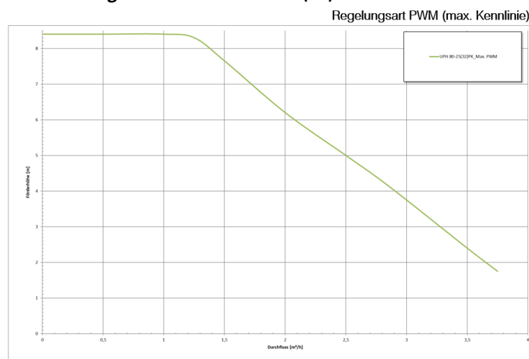
248 Abbildung: Kennlinien UPE 80-25(32) PK
