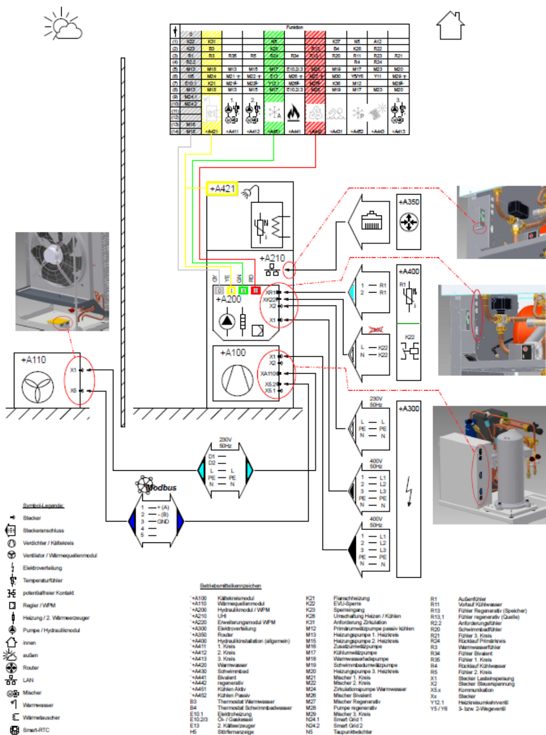
69 Abbildung: Anschlussplan System M Compact (230V)
