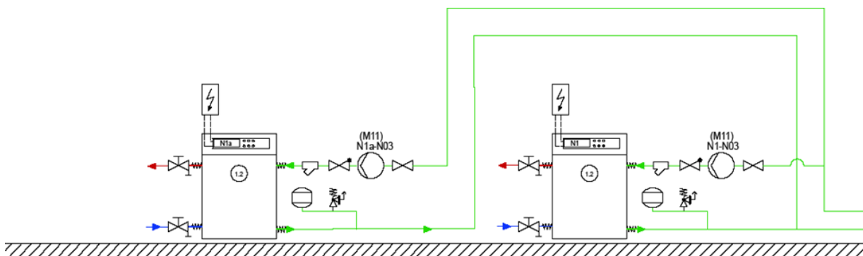
75 Abbildung: Parallelschaltung von Sole/Wasser-Wärmepumpen
