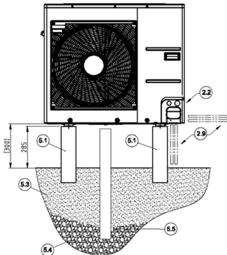
62 Abbildung: Fundamentplan LIA-Wärmepumpen mit kontrolliertem Ablauf
