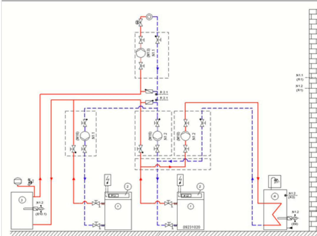
223 Abbildung: Einbindungsschema für die Parallelschaltung von Wärmepumpen, Reihen-Pufferspeicher mit einem doppelt-differenzdrucklosen Verteiler und Warmwasserbereitung
