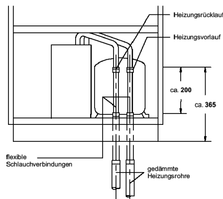
99 Abbildung: Einbindungsbeispiel einer Wärmepumpe für Außenaufstellung
