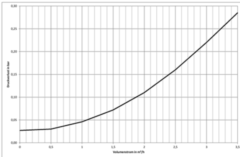
158 Abbildung: Druckverlust KPV 25 in Abhängigkeit des Volumenstroms
