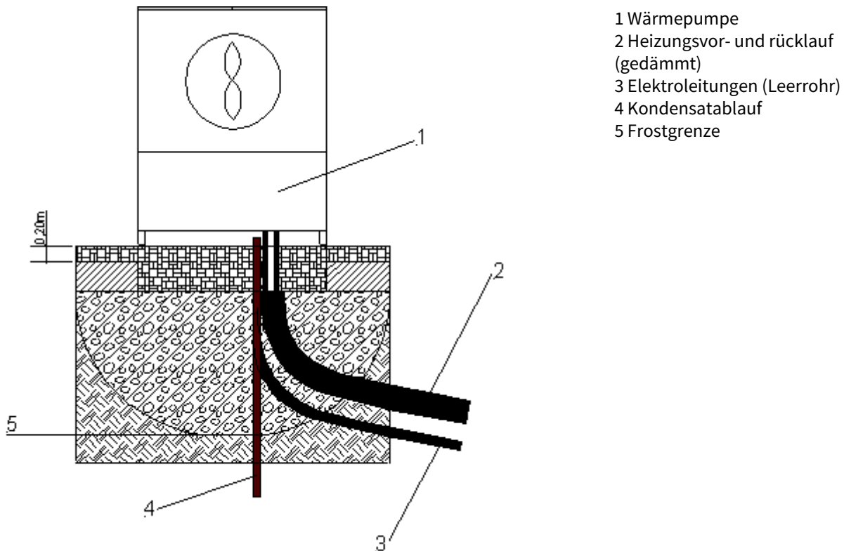
10 Abbildung: Fundamentplan Wärmepumpe mit Kondensatablauf
