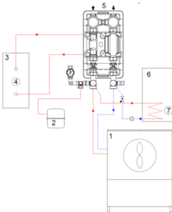
157 Abbildung: Einbindung des Kompaktverteilers für Heizbetrieb und Warmwasserbereitung
