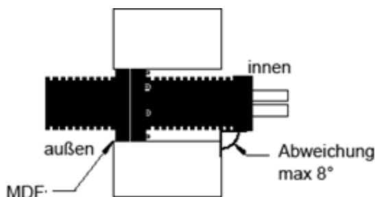
23 Abbildung: Skizze Mauerdurchführung drückendes Wasser
