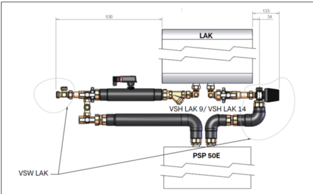
66 Abbildung: Verbindungssets Hydraulik (VSH LIA Flex) und Warmwasser (VSW LAK)
