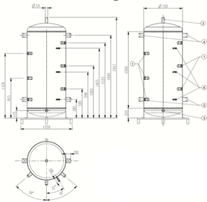
181 Abbildung: Abmessungen Pufferspeicher PSW 1000
