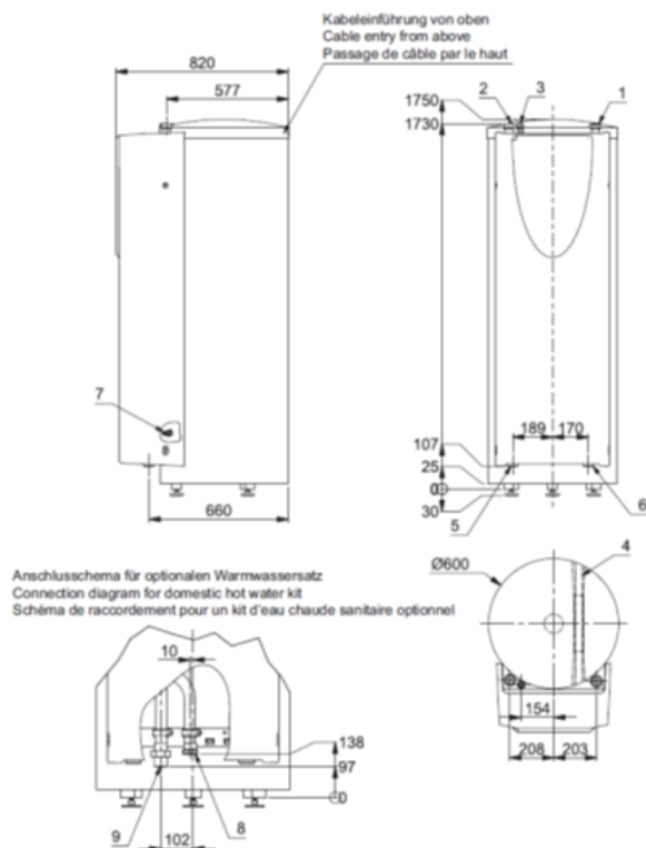
170 Abbildung: Aufbau Hydraulik-Tower HPK 300
