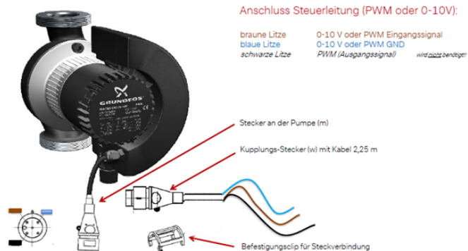
271 Abbildung: Elektrischer Anschluss Steuerskabel UPH 100-25(32) P und UPH 100-25(32) V
