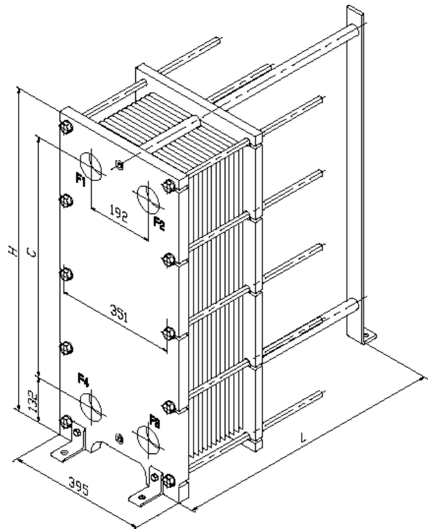
91 Abbildung: WTE 130
