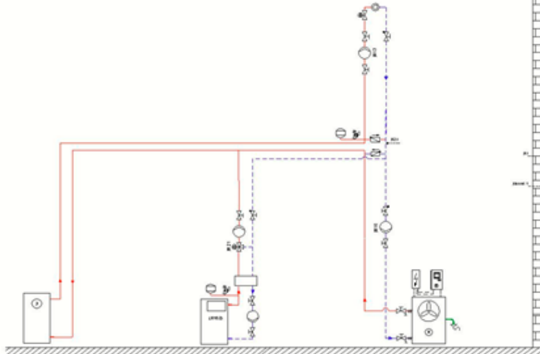
208 Abbildung: Einbindungsschema für den bivalenten Wärmepumpenbetrieb mit parallel eingebundenen Wärmeerzeuger
