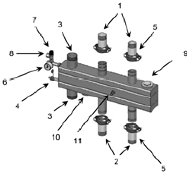
162 Abbildung: Doppelt differenzdrucklosen Verteiler DDV zum Anschluss eines gemischten Heizkreises, externer Heizungsunterstützung und optionaler Warmwasserbereitung.
