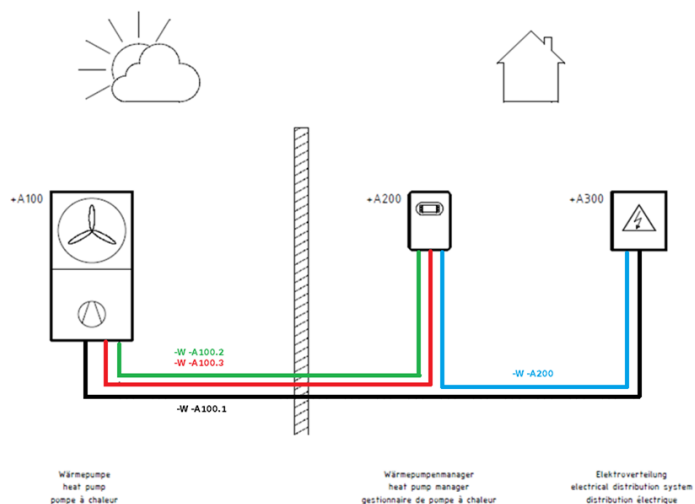
72 Abbildung: Kabelzugplan Luft/Wasser-Wärmepumpen für Außenaufstellung
