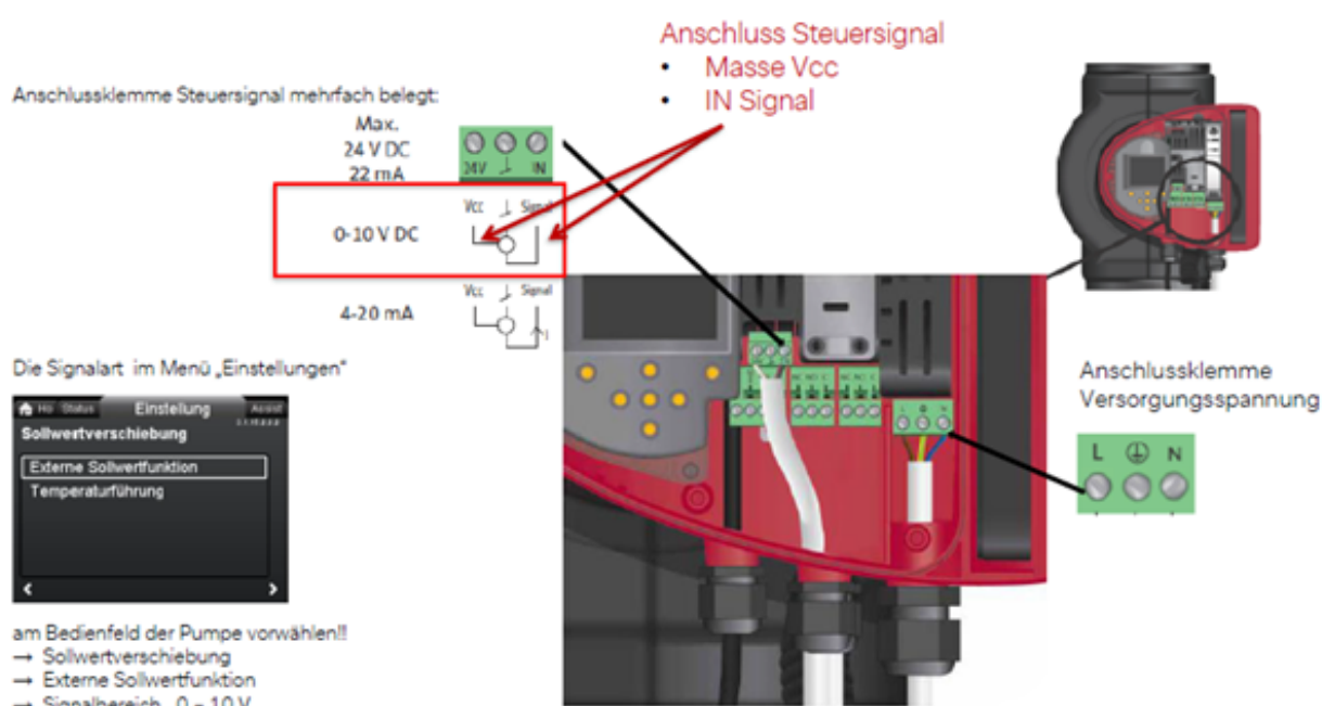
322 Abbildung: Elektrischer Anschluss Last (230 V) und Steuersignal Magna3-Baureihe
