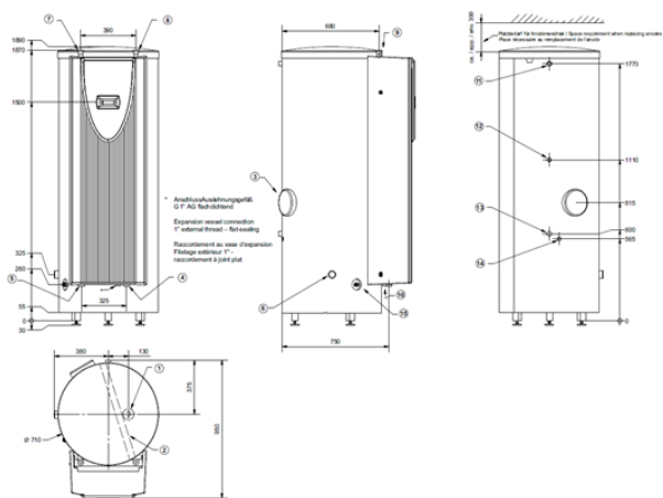
166 Abbildung: Aufbau Hydro-Tower HWK 332Econ(5S)
