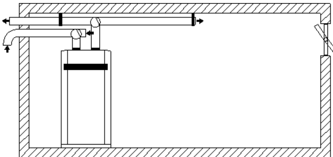
126 Abbildung: Variable Umschaltung der Ansaugluft
