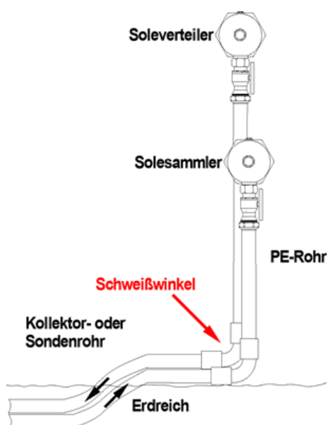
79 Abbildung: Montage der Rohrleitungen mit Schweißwinkel am Soleverteiler
