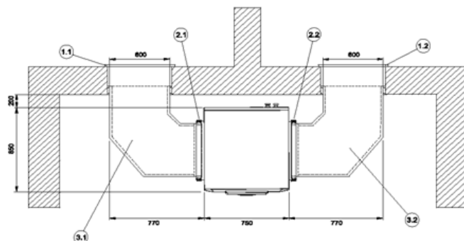
31 Abbildung: Wandaufstellung mit Luftkanal an der Ansaug- und Ausblasseite - Draufsicht
