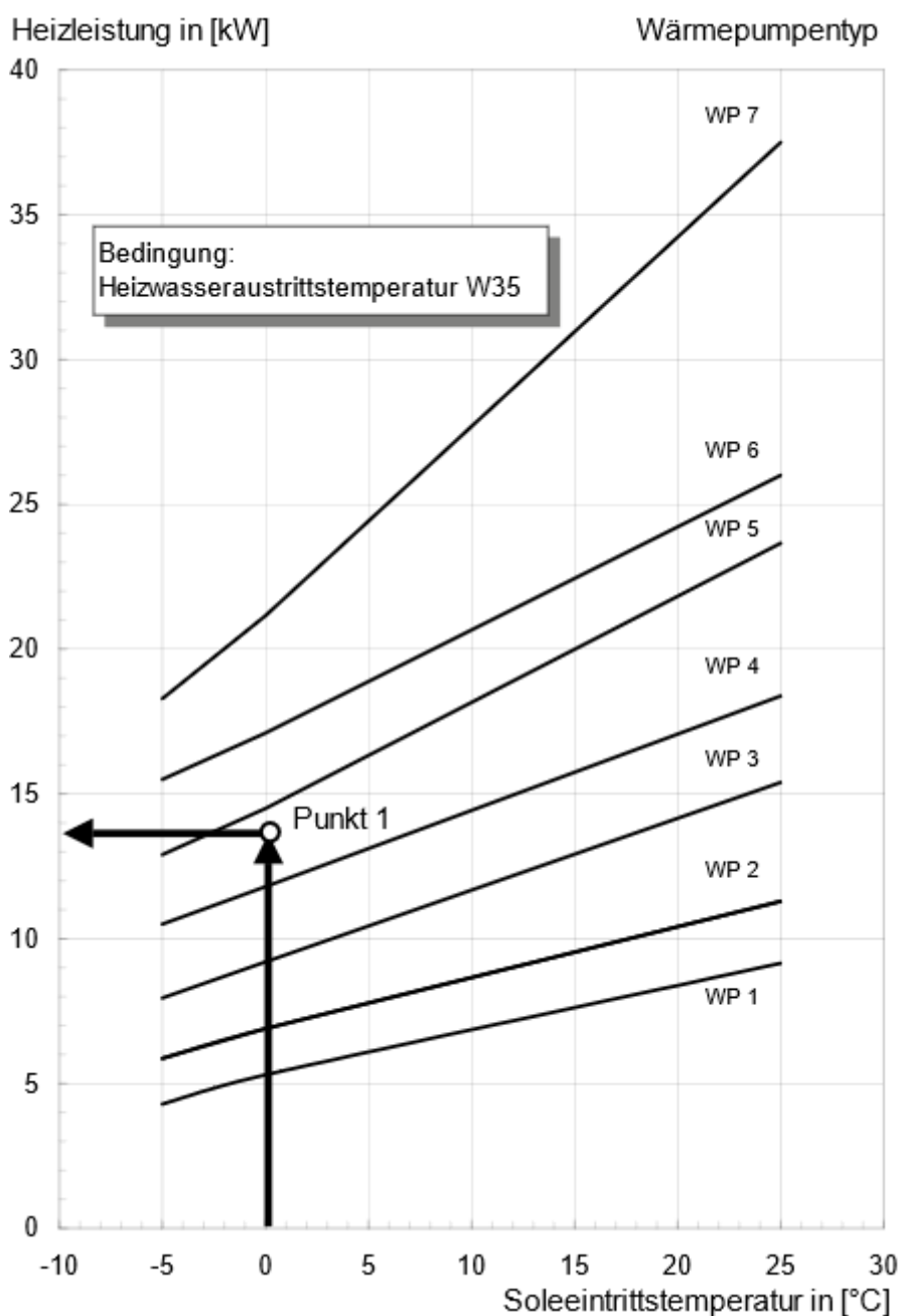
7 Abbildung: Heizleistungskurven von Sole//Wasser-Wärmepumpen unterschiedlicher Heizleistungen für Vorlauftemperaturen von 35 °C
