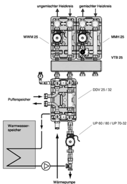
160 Abbildung: Einbindung des doppelt differenzdruckloser Verteilers für Heizbetrieb und Warmwasserbereitung
