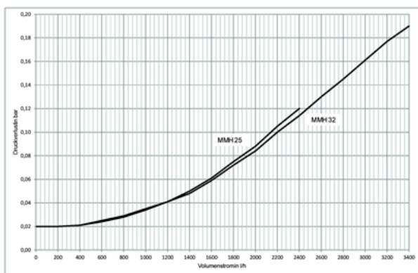
148 Abbildung: Diagramm Druckverlust MMH 25 und MMH 32
