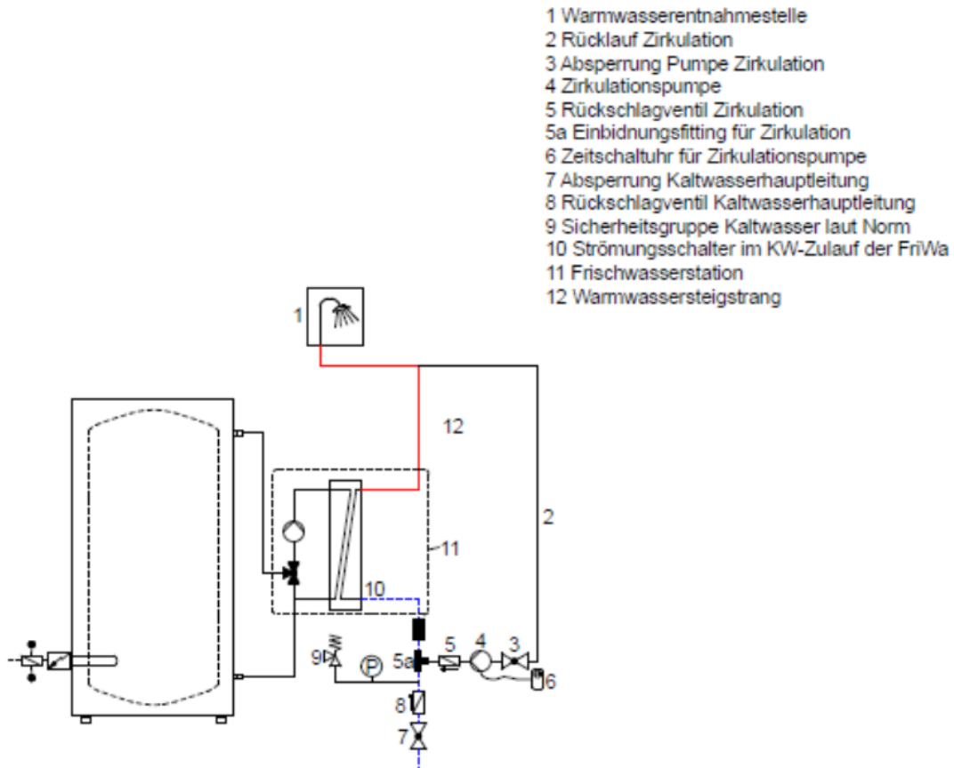
119 Abbildung: Funktionsschema Frischwasserstation mit Zirkulationsanschluss
