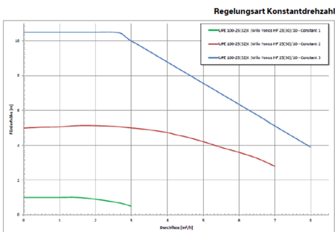
254 Abbildung: Kennlinien UPE 100-25(32)K
