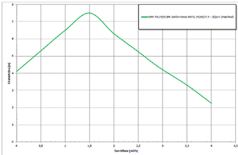
245 Abbildung: Kennlinien UPE 70-25(32)PK
