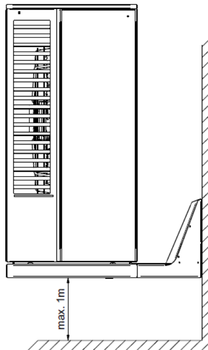
60 Abbildung: Aufstellung Außeneinheit M Flex und System M mit Wandkonsole
