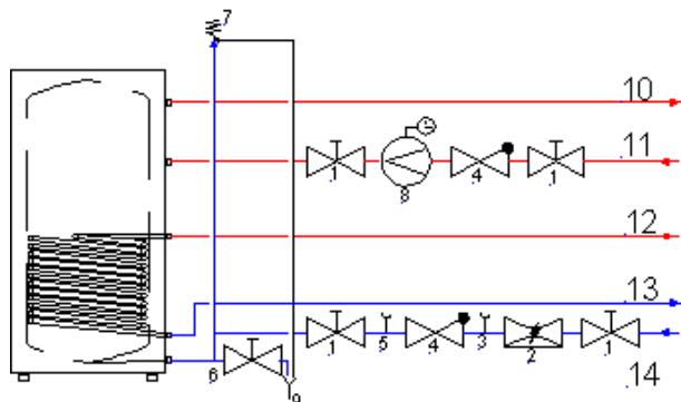
107 Abbildung: Wasserseitiger Anschluss
