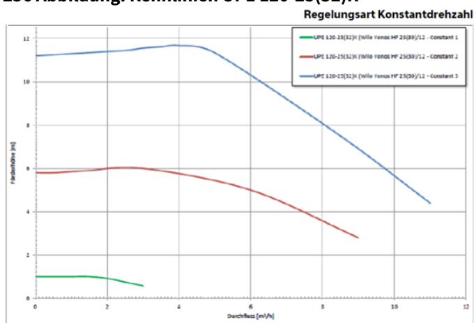
257 Abbildung: Kennlinien UPE 120-25(32)K
