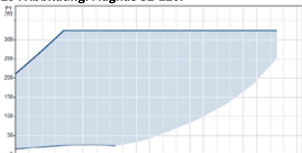
295 Abbildung: Leistungsaufnahme Magna3 32-120F
