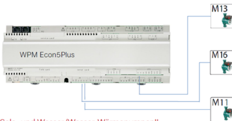
287 Abbildung: Elektrische Verdrahtung Steuersignal 0 - 10V und PWM für Sole/Wasser-Wärmepumpen am WPM Econ5Plus
