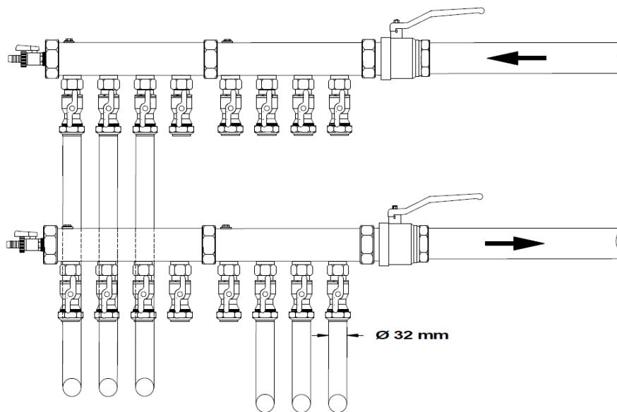
76 Abbildung: Montage Soleverteiler bis max. 8 Kreise
