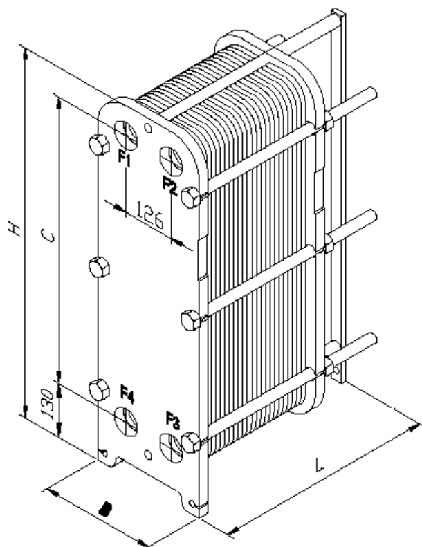
93 Abbildung: WTE 40
