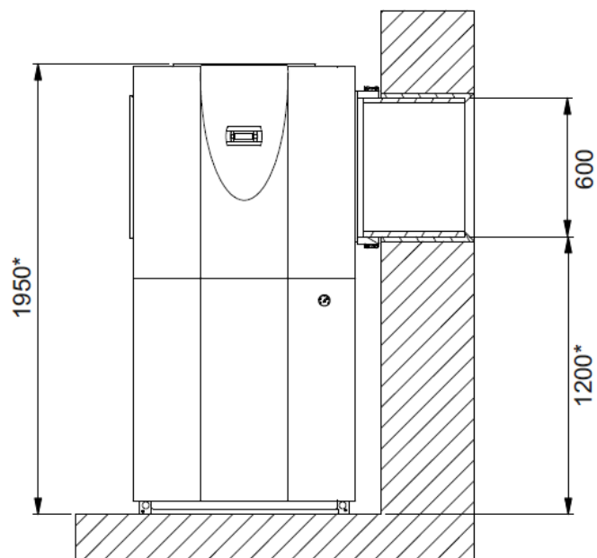
48 Abbildung: Frontansicht - LIK 12TU (Eck-Aufstellung) LIK 12TU - Wand-Aufstellung mit Luftkanal auf der Ausblasseite
