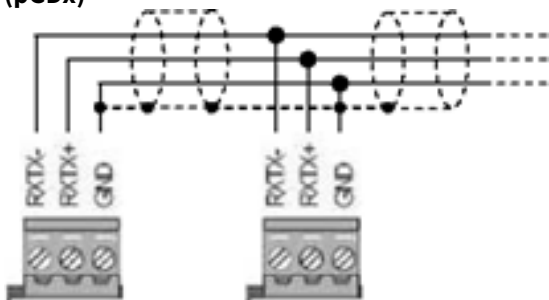
138 Abbildung: Ansicht des Anschlusses an der Klemme J11 des WPM
