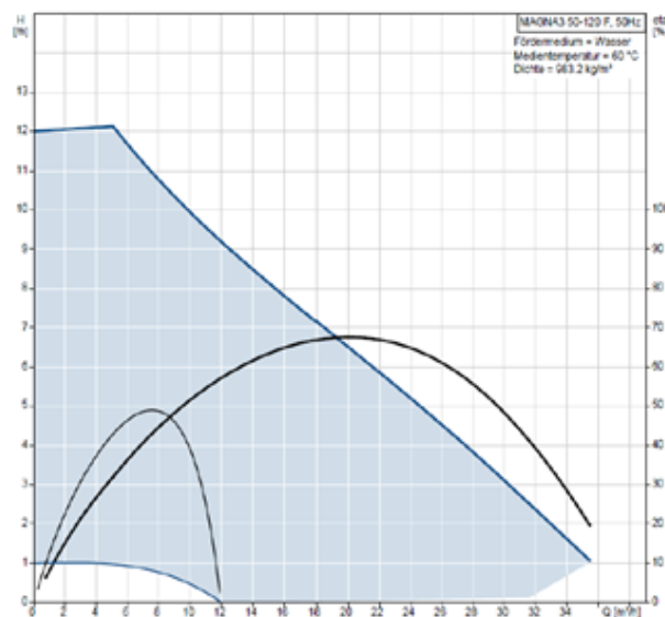
305 Abbildung: Förderhöhe Magna3 50-120F
