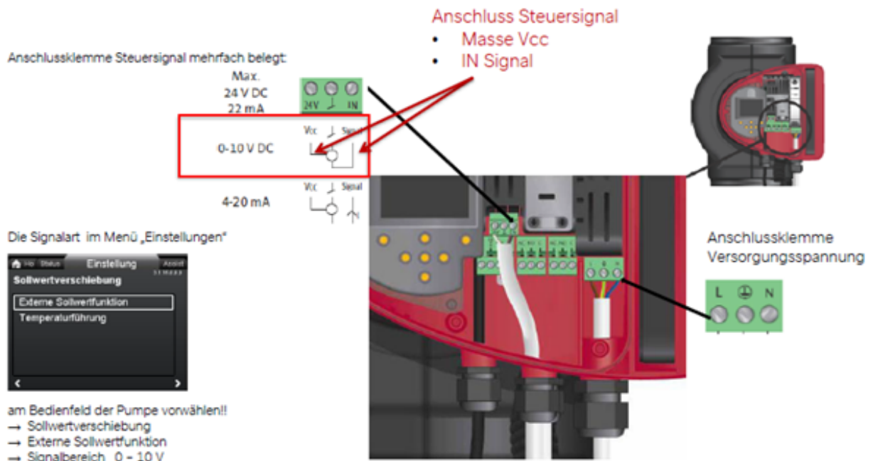
282 Abbildung: Elektrischer Anschluss UPH 80-40F und UPH 120-50F
