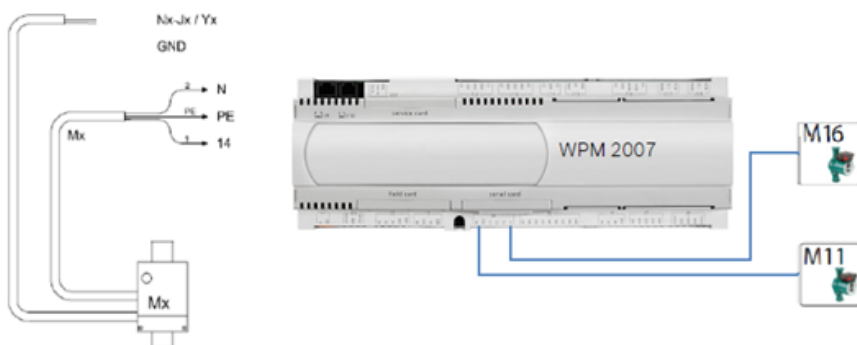
284 Abbildung: Elektrische Verdrahtung Steuersignal 0 - 10V am WPM 2006/2007Plus
