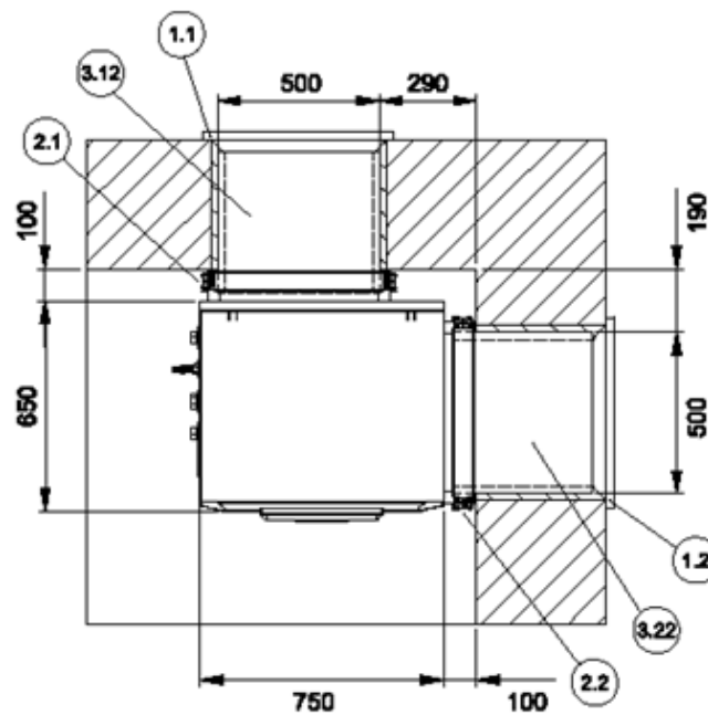
37 Abbildung: Draufsicht - LIK 8TES (Eck-Aufstellung)
