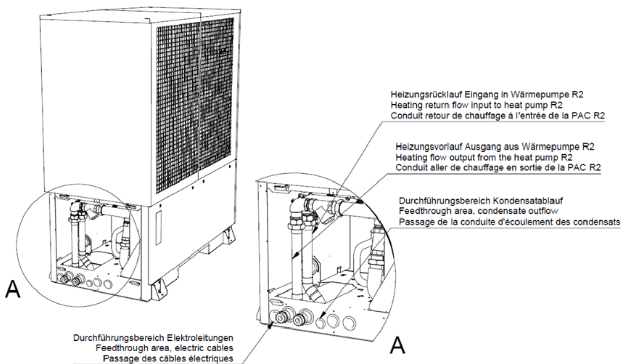
20 Abbildung: Hydraulische und elektrische Anschlüsse bei seitlichem Anschluss
