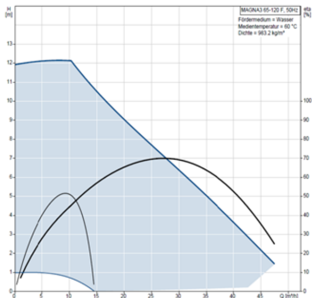
314 Abbildung: Förderhöhe Magna3 65-120F
