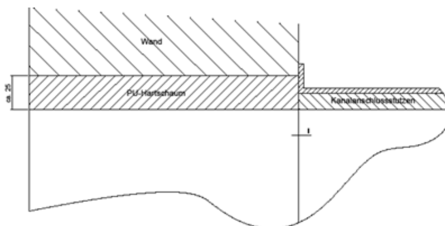
28 Abbildung: Beispiel für die Ausführung eines Mauerdurchbruches
