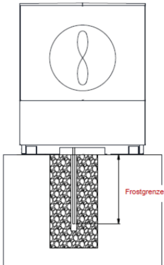
11 Abbildung: Kondensatablauf in Kiesschüttung
