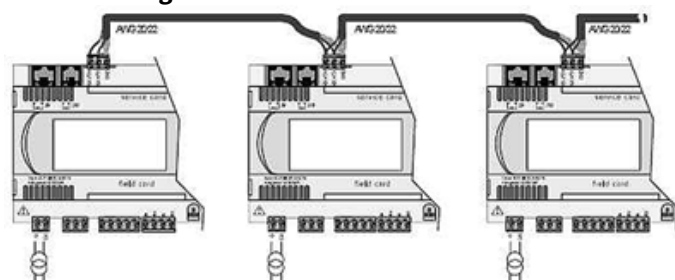
139 Abbildung: Drei Wärmepumpenmanager mit jeweils eigener Spannungsversorgung
