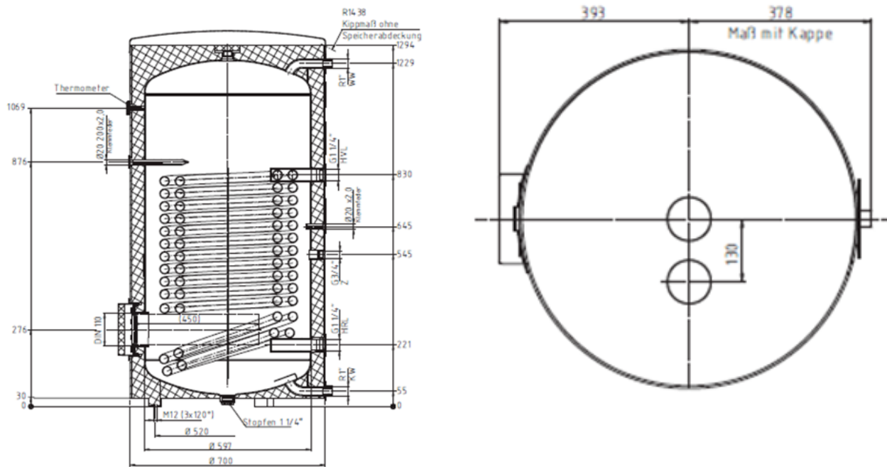
113 Abbildung: Zeichnung WWSP 335
