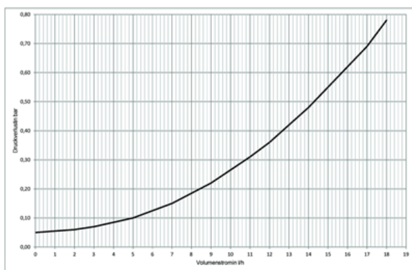
151 Abbildung: Diagramm Druckverlust WMM 50
