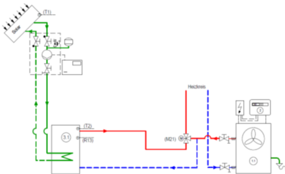
185 Abbildung: 3-Wege-Mischer für den bivalenten Betrieb der Wärmepumpe (Schaltbeispiel für den Heizbetrieb mit einer Solarthermieanlage)
