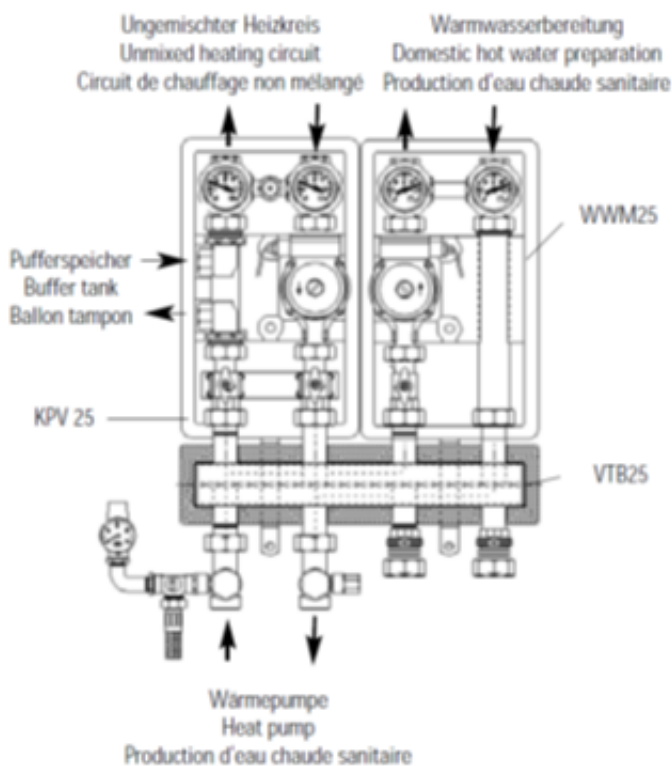
155 Abbildung: Kompaktverteiler KPV 25 mit Verteilerbalken VTB 25 und Warmwassermodul WWM 25
