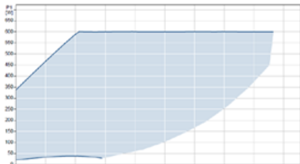
310 Abbildung: Leistungsaufnahme Magna3 65-100F
