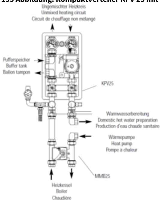
156 Abbildung: Kompaktverteiler KPV 25 mit Mischer-Modul bivalent MMB 25
