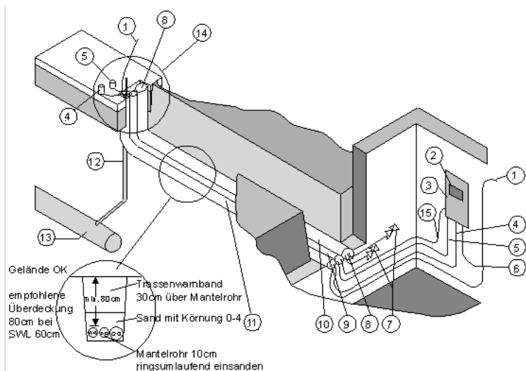
19 Abbildung: Hydraulische und elektrische Anschlüsse bei Erdverlegung
