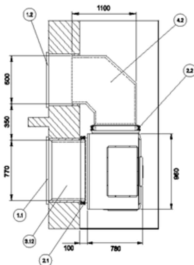
30 Abbildung: Wandaufstellung mit Luftkanal Ausblasseite - Draufsicht
