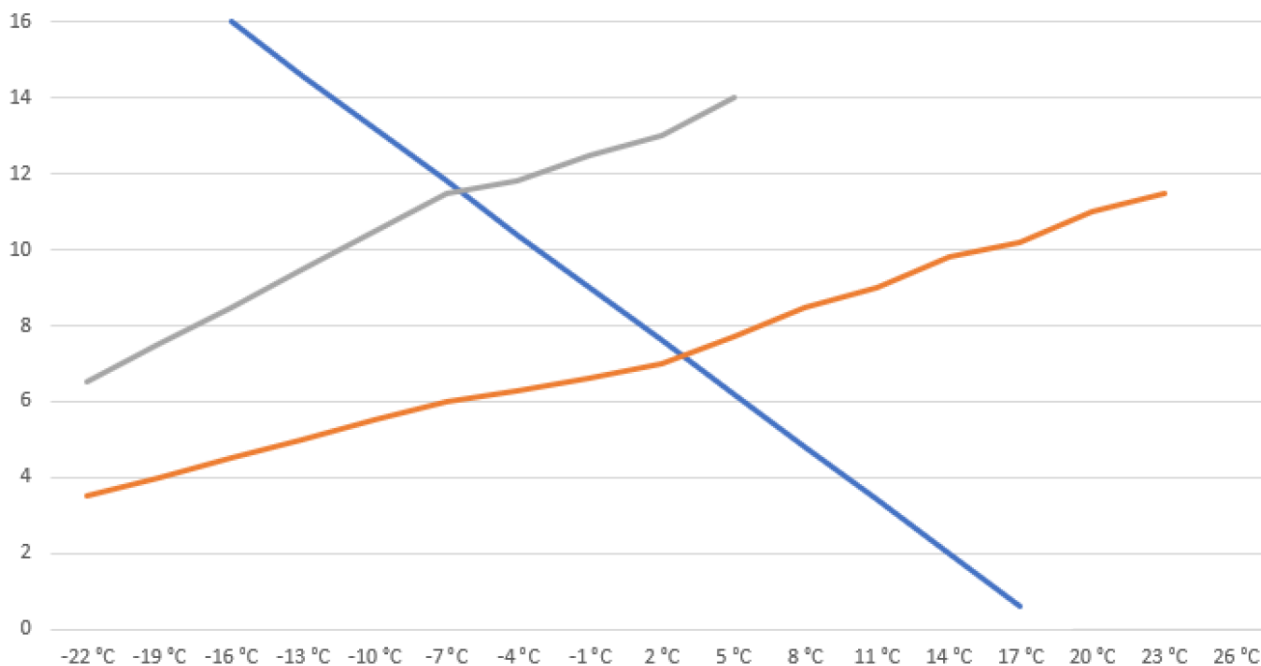
3 Abbildung: Heizleistungskurven Wärmepumpen mit zwei Leistungsstufen (stufige Regelung)
