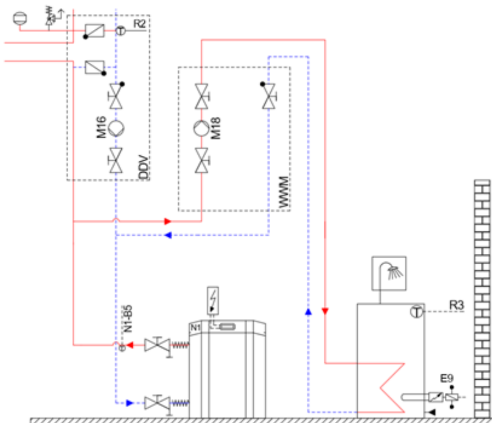
190 Abbildung: Warmwasserbereitung über Umwälzpumpe M 18 mit Rückschlagklappen im Erzeuger- und Warmwasserkreis
