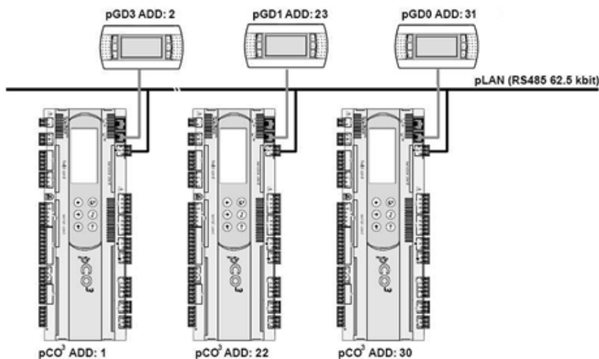
137 Abbildung: Beispiel eines möglichen Netzwerks inkl. drei Wärmepumpenmanager mit 3 Bedienteilen (pGDx)
