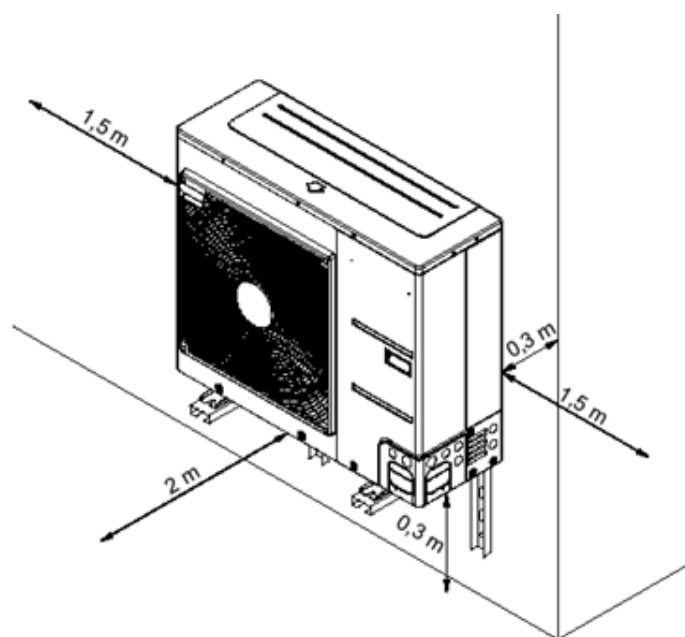
58 Abbildung: Aufstellung Außeneinheit LAW 9IMR mittels Wandkonsole
