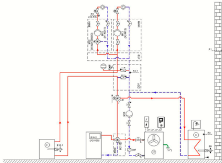
209 Abbildung: Einbindungsschema für den bivalenten Wärmepumpenbetrieb mit Heizkessel, zwei Heizkreisen, Reihen-Pufferspeicher und Warmwasserbereitung.
