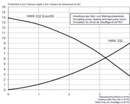
167 Abbildung: Pumpen-, Gerätekenlinie Heiz- und Wärmepumpenkreis HWK 332Econ(5S)
