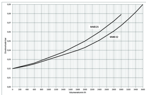
147 Abbildung: Diagramm Druckverluste MMB 25 und MMB 32
