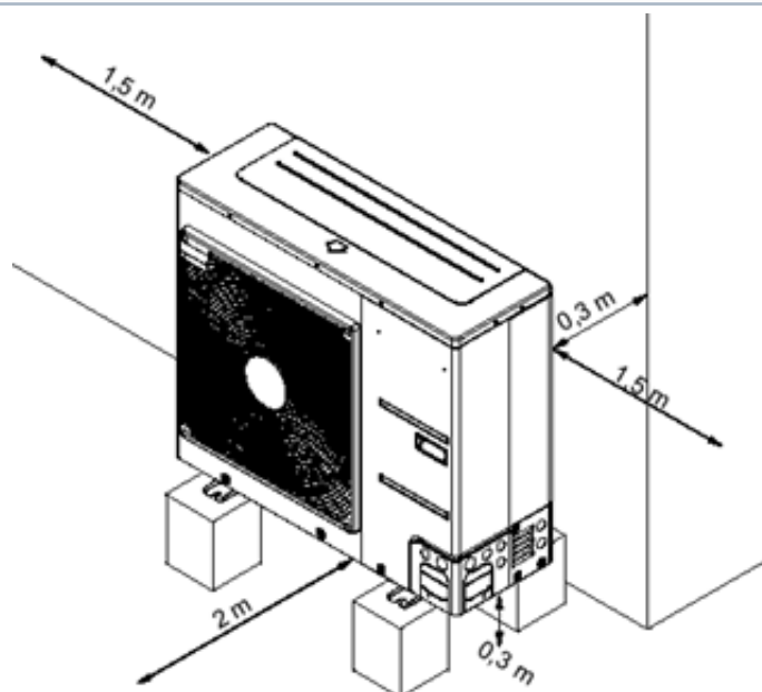
57 Abbildung: Aufstellung Außeneinheit LAW 9IMR
