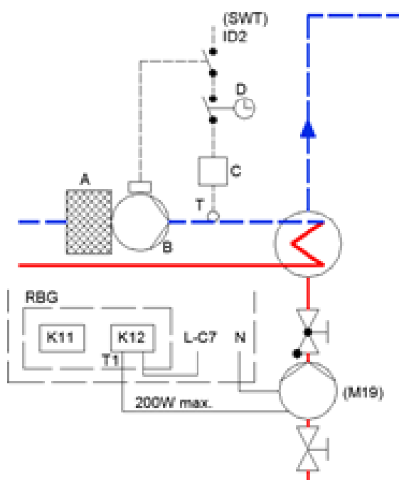
188 Abbildung: Einbindung für die Schwimmbadwasser-Erwärmung mit Wärmepumpen mit Relaisbaugruppe
