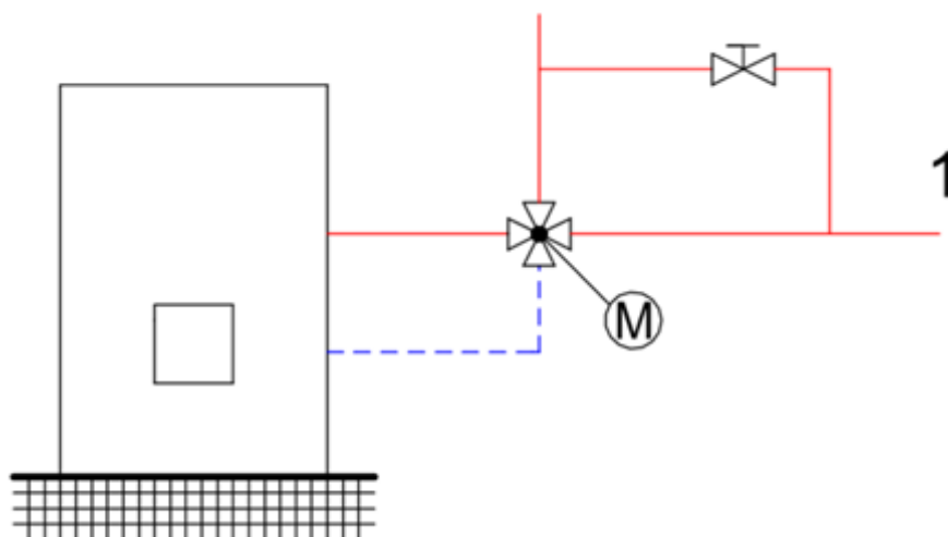
183 Abbildung: Bypass-Schaltung zur Absicherung der maximalen Vorlauftemperatur
