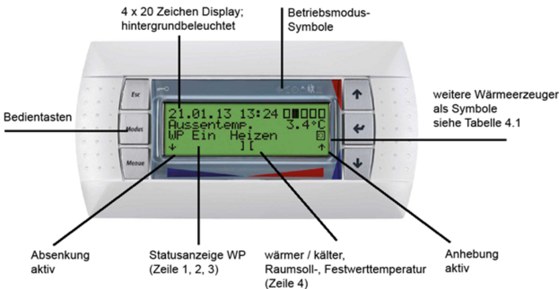
131 Abbildung: Wärmepumpenmanager WPM 2007 plus bzw. WPM EconPlus mit abgesetztem LC-Display Standardanzeige mit Bedientasten
