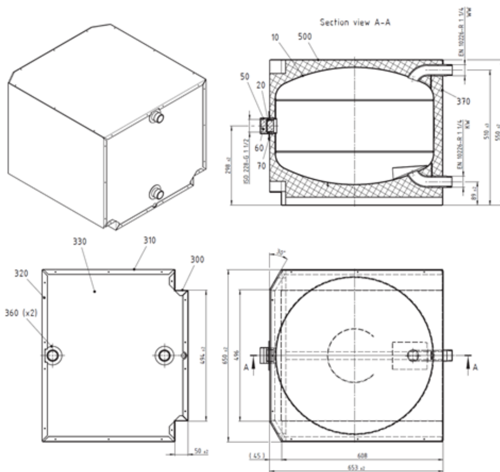
176 Abbildung: Abmessungen des Unterstell-Pufferspeichers PSP 100U für die Sole/Kompakt-Wärmepumpe
