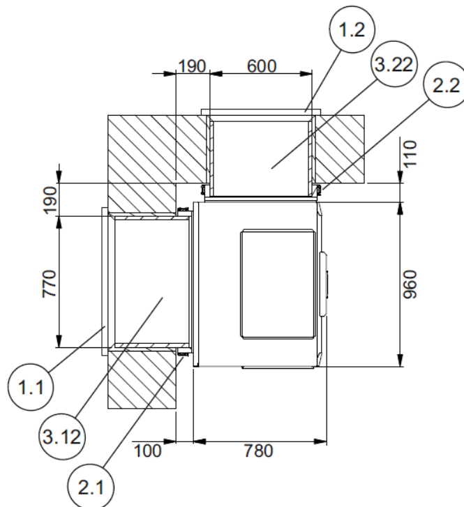
47 Abbildung: Draufsicht - LIK 12TU (Eck-Aufstellung)
