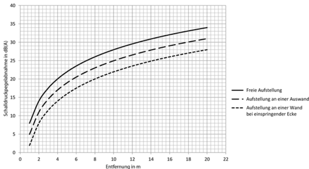
98 Abbildung: Schalldruckpegelabnahme bei unterschiedlicher Aufstellung
