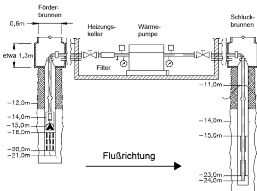
89 Abbildung: Beispiel einer Einbindung der Wasser/Wasser-Wärmepumpe mit Förder- u. Schluckbrunnen
