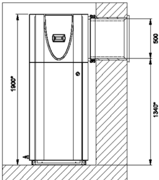
38 Abbildung: Frontansicht - LIK 8TES (Eck-Aufstellung)
