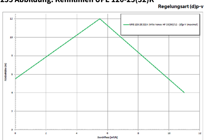
256 Abbildung: Kennlinien UPE 120-25(32)K
