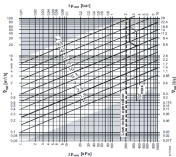
151 Abbildung: Diagramm Druckverlust WMM 50
