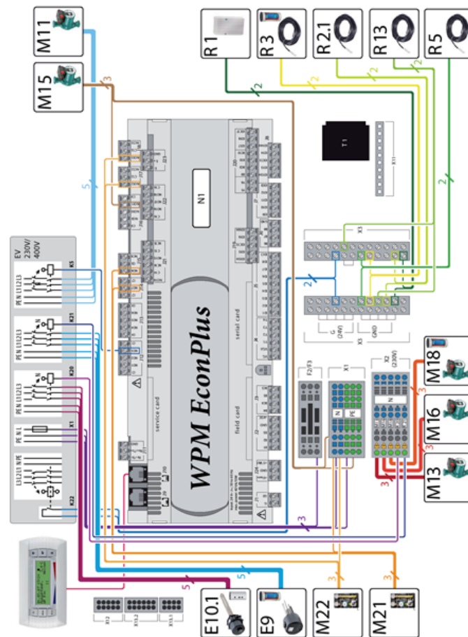
213 Abbildung: Anschlussplan Wärmepumpenmanager WPM EconPlus bei bivalent regenerativen Anlagen mit zwei Heizkreisen und Warmwasserbereitung.
