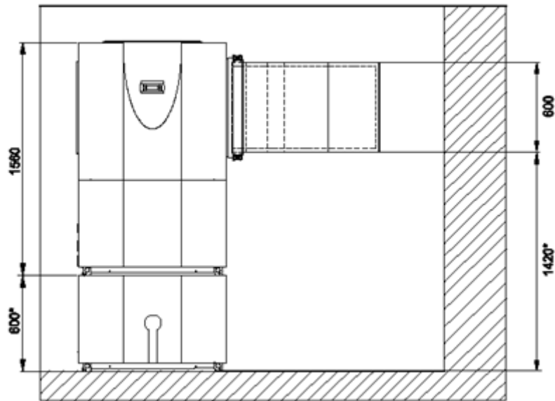
35 Abbildung: Frontansicht - LI 12TU und LI 16I-TUR (Wand-Aufstellung – Luftkanal Ausblasseite)
