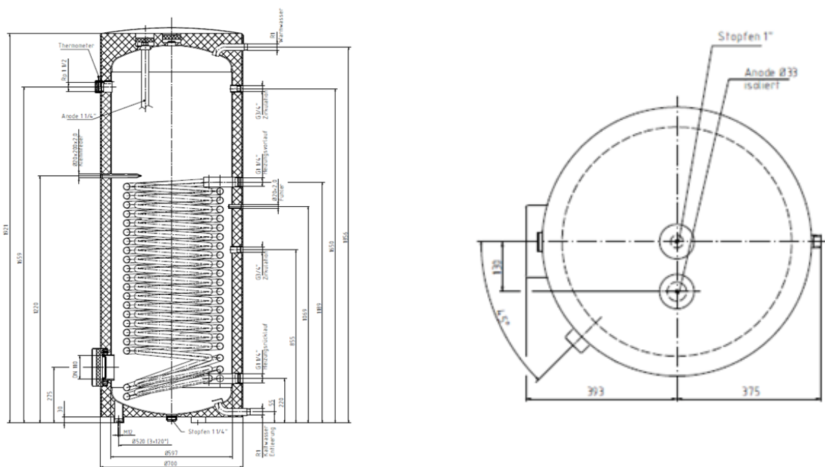
115 Abbildung: Zeichnung WWSP 556
