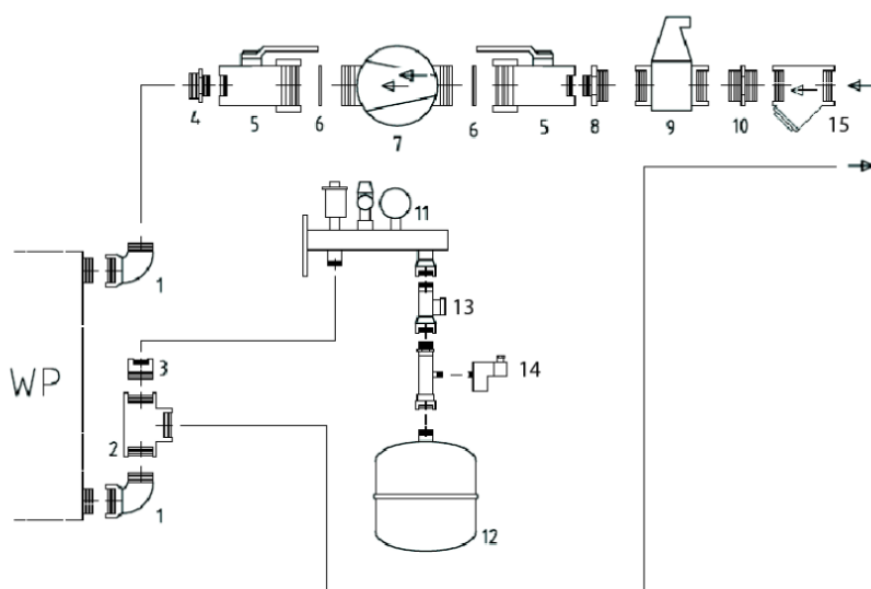
81 Abbildung: Aufbau Solekreisleitung inkl. Einbauten
