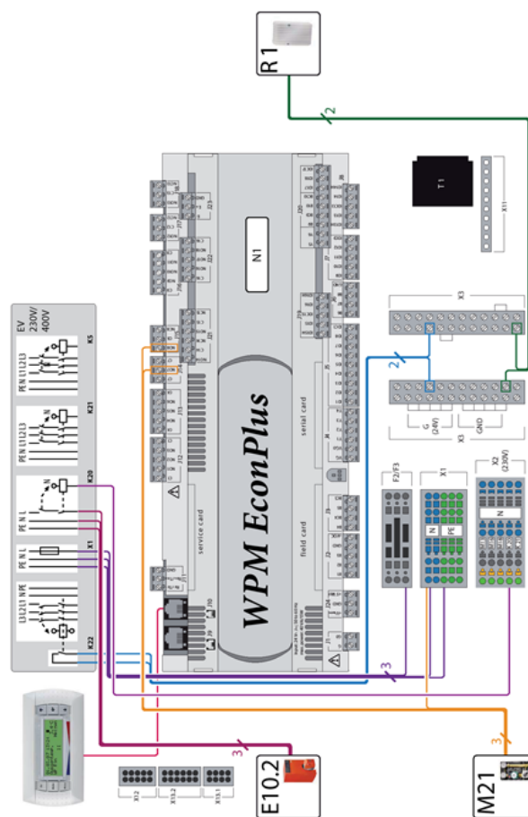
201 Abbildung: Anschlussplan Wärmepumpenmanager WPM EconPlus bei bivalenten Anlagen mit Hydro-Tower HWK 332
