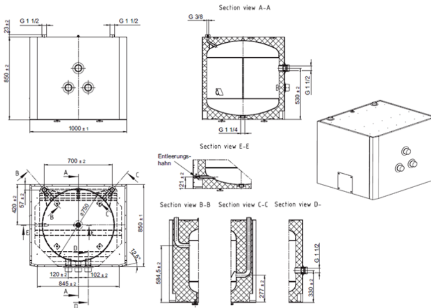
178 Abbildung: Abmessungen des Unterstell-Pufferspeichers PSP 300U
