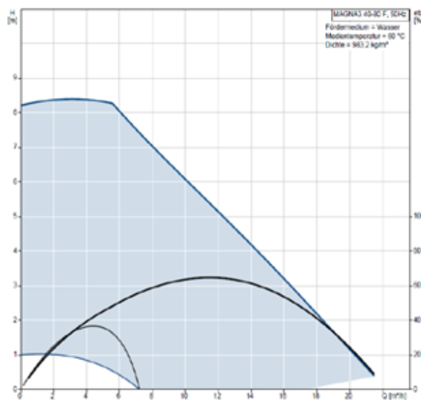
278 Abbildung: Einsatzgrenzen und Kennlinien UPH 80-40F
