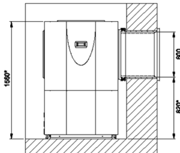
43 Abbildung: Frontansicht - LI 12TU und LI 16I-TUR (Eck-Aufstellung) LI 9TU, LI 12TU und LI 16I-TUR - Wand-Aufstellung mit Luftkanal auf der Ausblasseite
