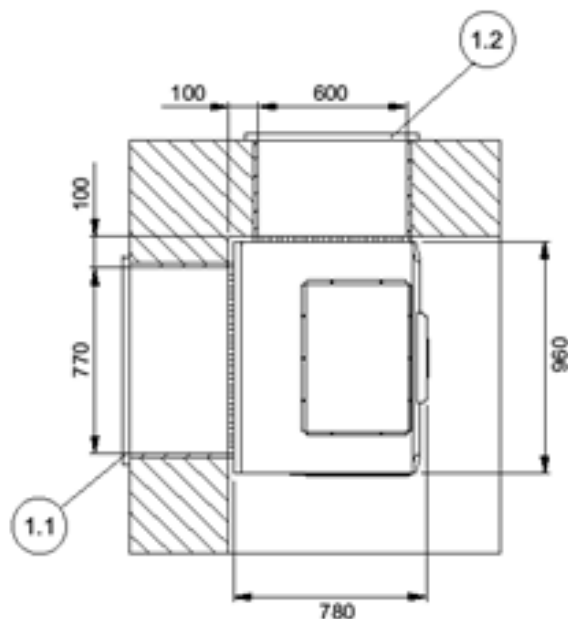
29 Abbildung: Draufsicht - direkte Eckaufstellung mit Dämmstreifen
