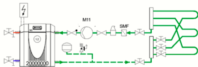
191 Abbildung: Schematische Darstellung der Einbindung von Sole/Wasser-Wärmepumpen
