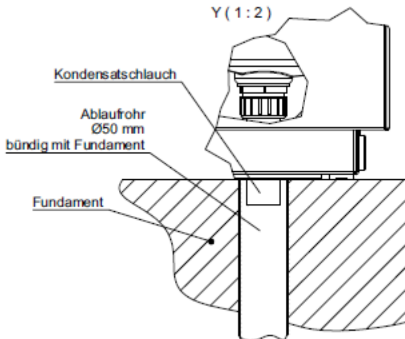
56 Abbildung: Kondensatablauf M Flex und System M
