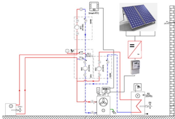
143 Abbildung: Einbindungsschema zur Nutzung variabler Tarife mit Reihen-Pufferspeicher und Warmwasserspeicher
