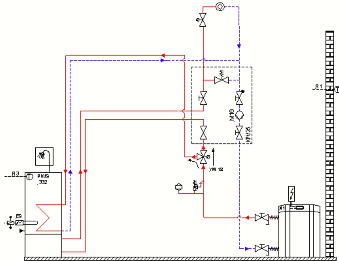
194 Abbildung: Einbindungsschema für den monovalenten Wärmepumpenbetrieb mit einem Heizkreis, Reihen-Pufferspeicher und Warmwasserbereitung.
