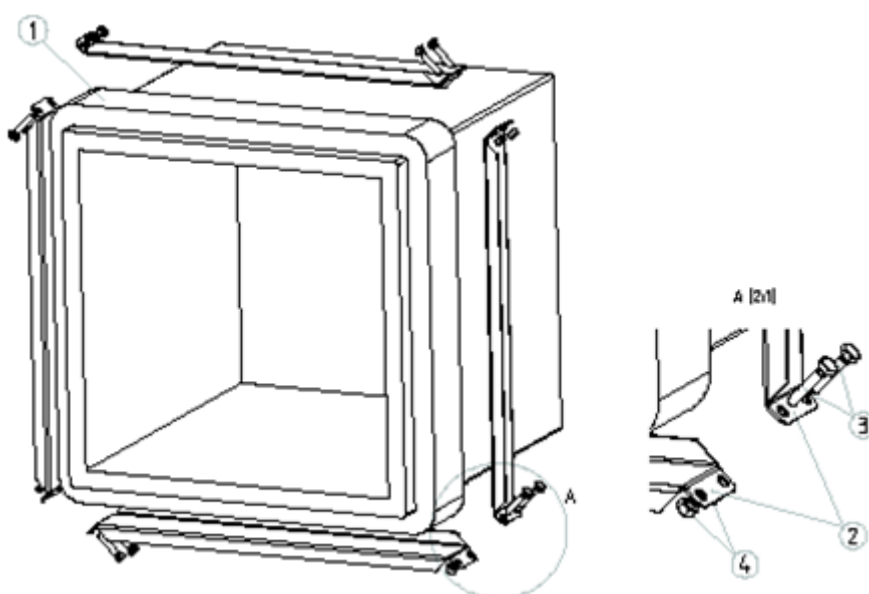
24 Abbildung: Dichtmanschette für Luftkanäle Regenschutzgitter für Wärmepumpen
