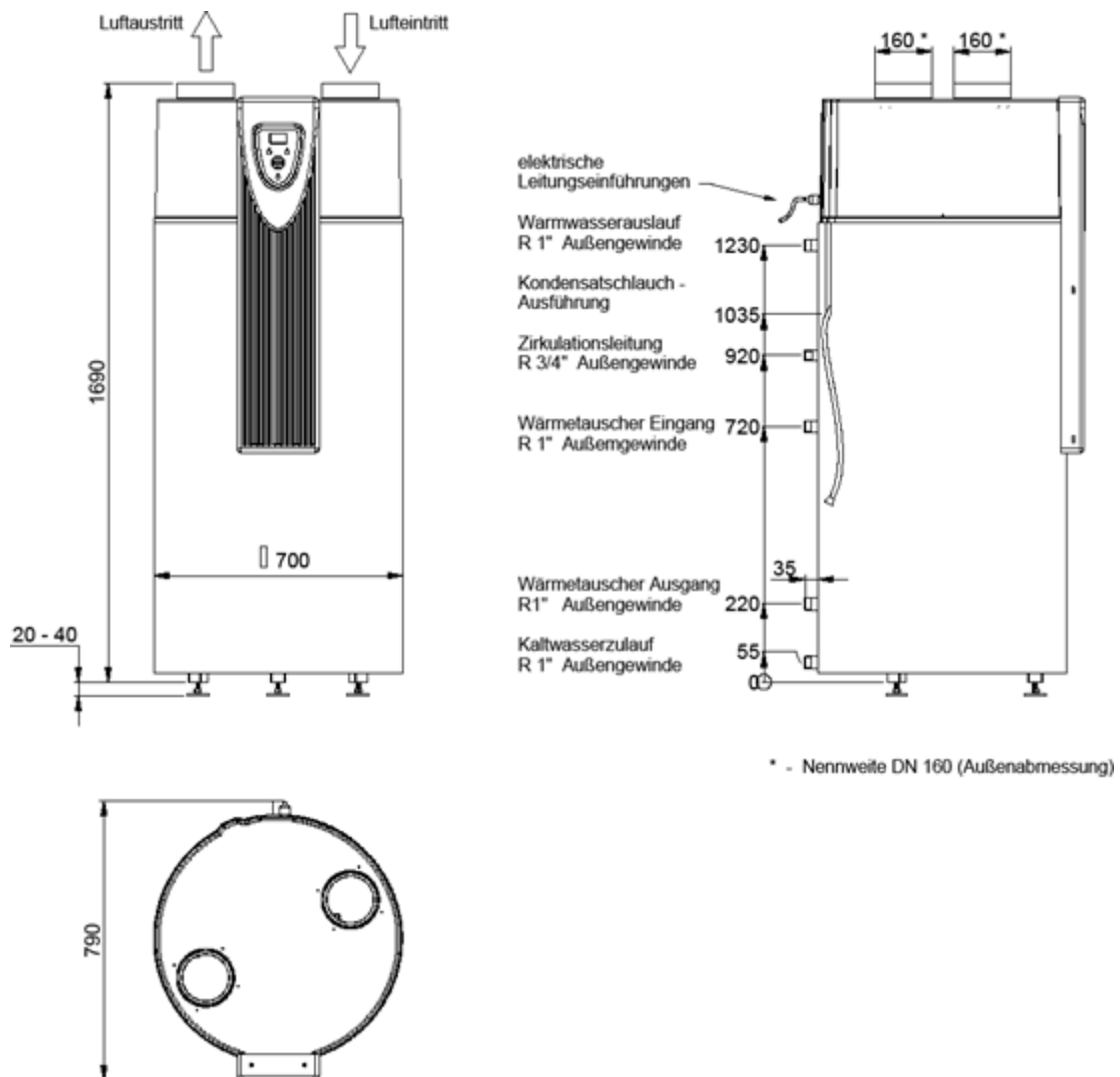
124 Abbildung: Anschlüsse und Abmaße einer Warmwasser-Wärmepumpe mit innen liegendem Zusatz-Wärmeübertrager
