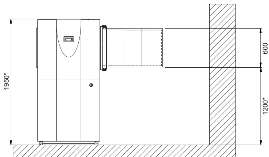
50 Abbildung: Frontansicht - LIK 12TU (Wand-Aufstellung mit Luftkanal auf der Ausblasseite)
