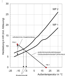
6 Abbildung: Heizleistungskurven von zwei Luft/Wasser-Wärmepumpen unterschiedlicher Heizleistungen für Vorlauftemperaturen von 35 °C und außentemperaturabhängigem Gebäudewärmebedarf
