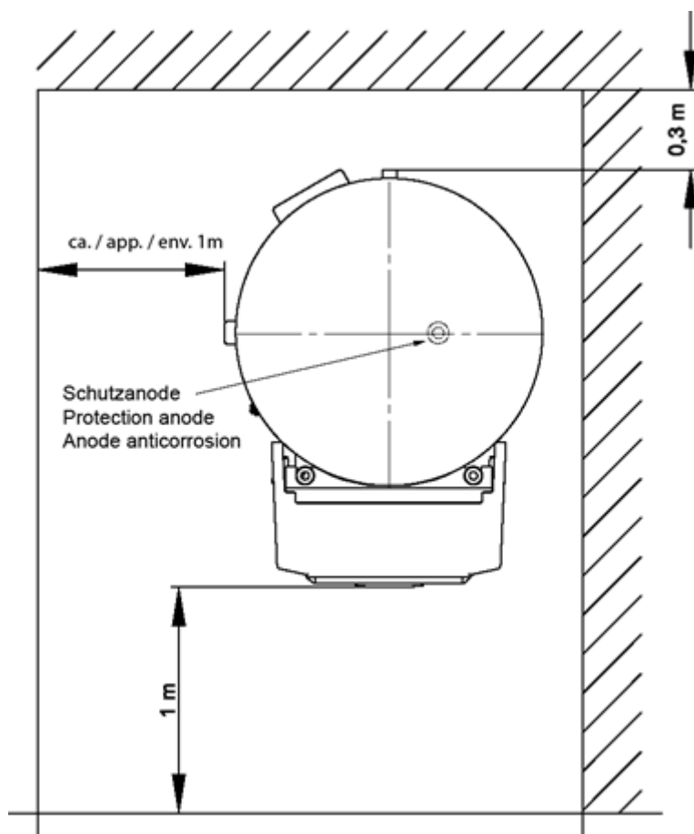
64 Abbildung: Aufstellung Inneneinheit LIA...BWCF (M)
