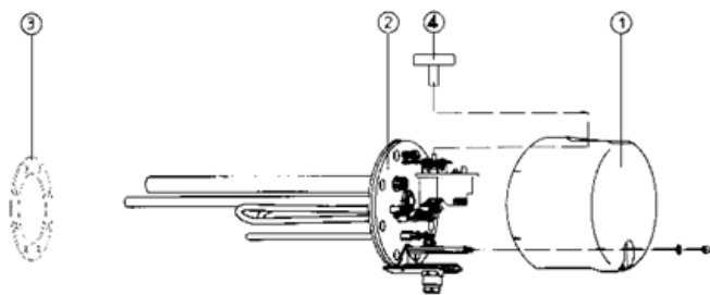
105 Abbildung: Aufbau einer Flanschheizung
