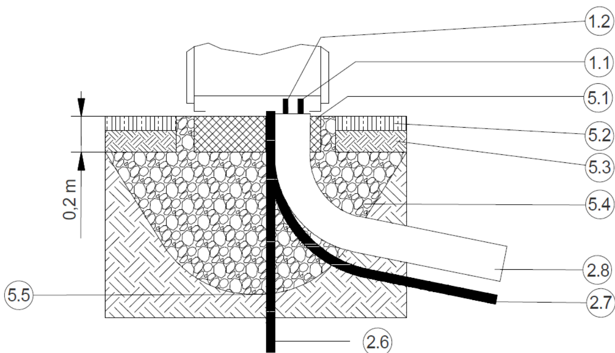
63 Abbildung: Fundamentplan M Flex und System M Comfort mit Kiesbett
