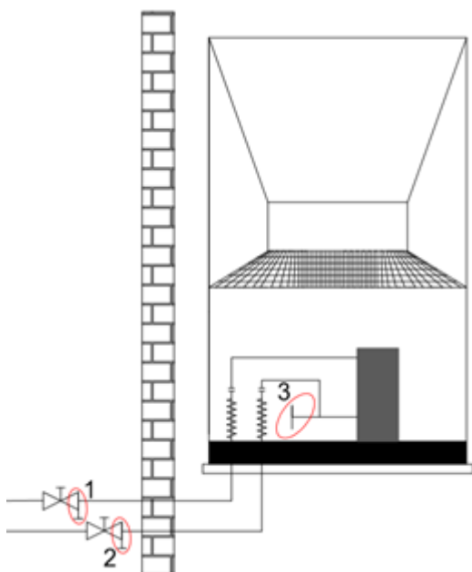
145 Abbildung: Schaltbild für die Installation von frostgefährdeten Wärmepumpen
