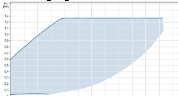
316 Abbildung: Leistungsaufnahme Magna3 65-150F
