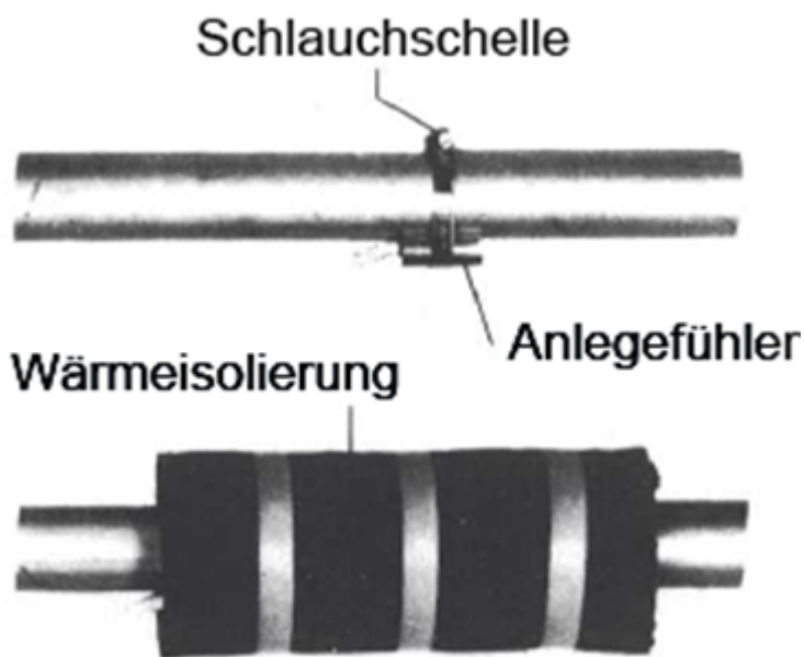
135 Abbildung: Montage eines Rohranlegefühlers
