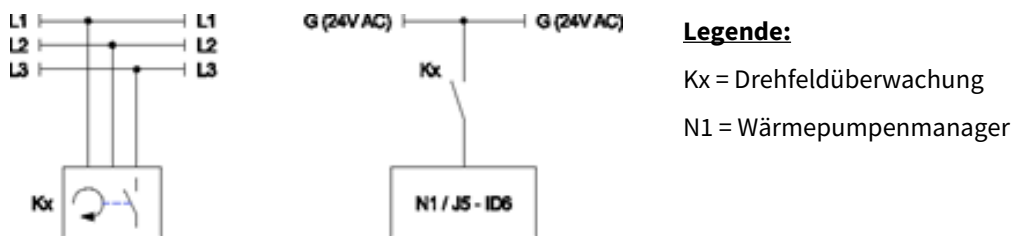
136 Abbildung: Anschluss Drehfeldüberwachung
