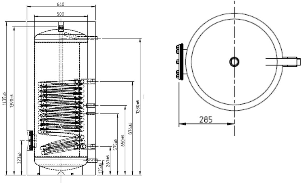
112 Abbildung: Zeichnung WWSP 229
