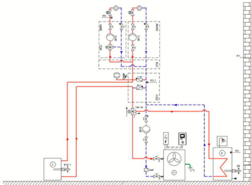
205 Abbildung: Einbindungsschema für den monoenergetischen Wärmepumpenbetrieb mit zwei Heizkreisen, Reihen-Pufferspeicher und Warmwasserbereitung
