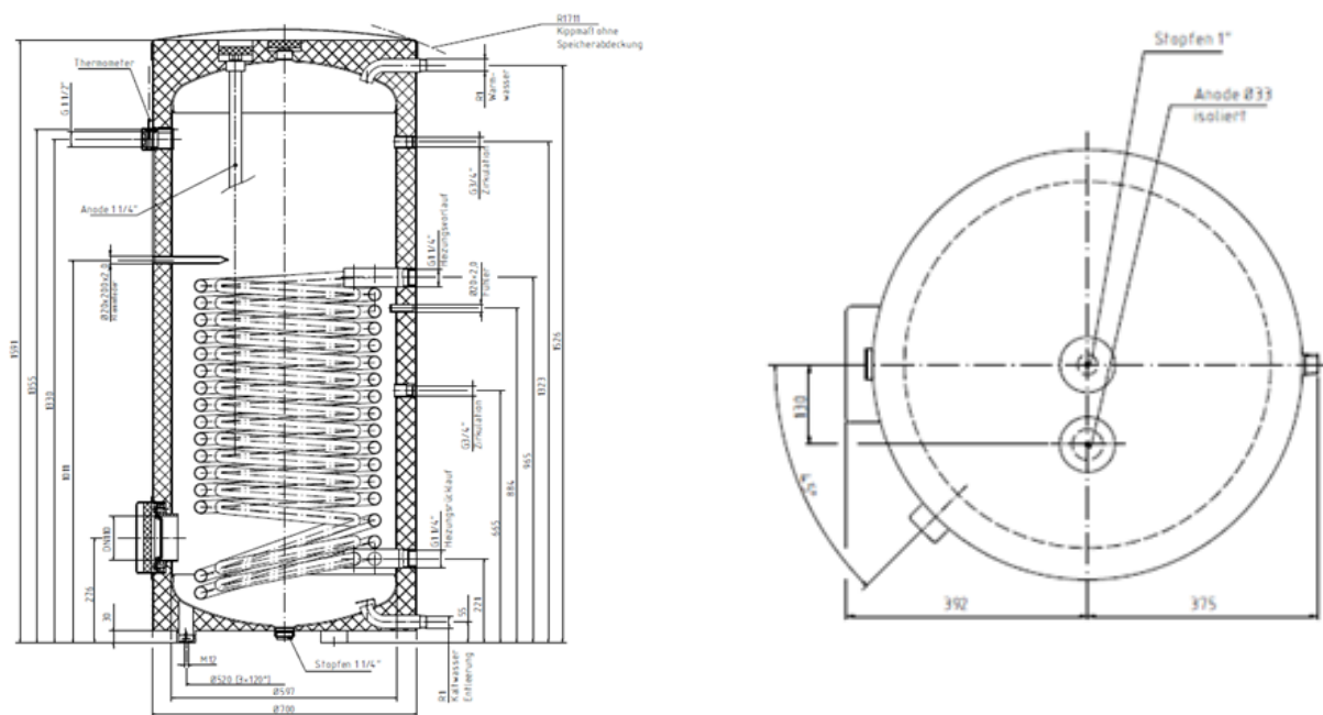
114 Abbildung: Zeichnung WWSP 442
