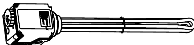
106 Abbildung: Aufbau des Einschraubheizkörpers CEHK
