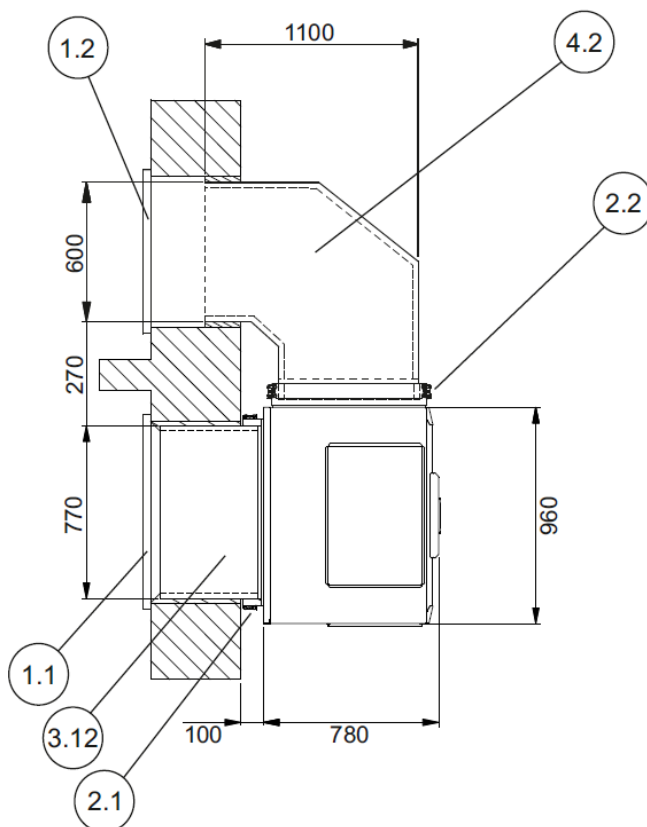
49 Abbildung: Draufsicht - LIK 12TU (Wand-Aufstellung mit Luftkanal auf der Ausblasseite)
