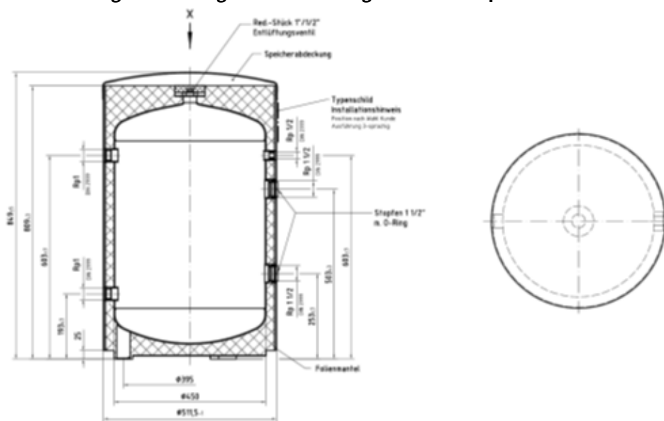
174 Abbildung: Abmessungen des wandhängenden Pufferspeichers PSP 50E
