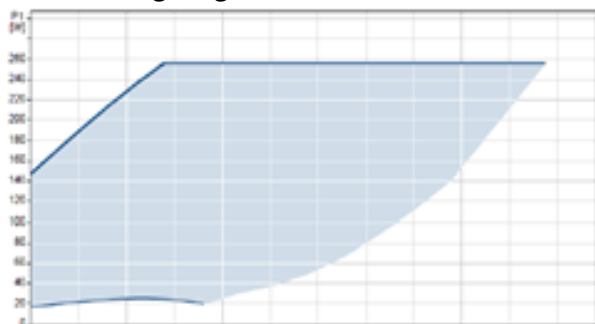
298 Abbildung: Leistungsaufnahme Magna3 40-80F
