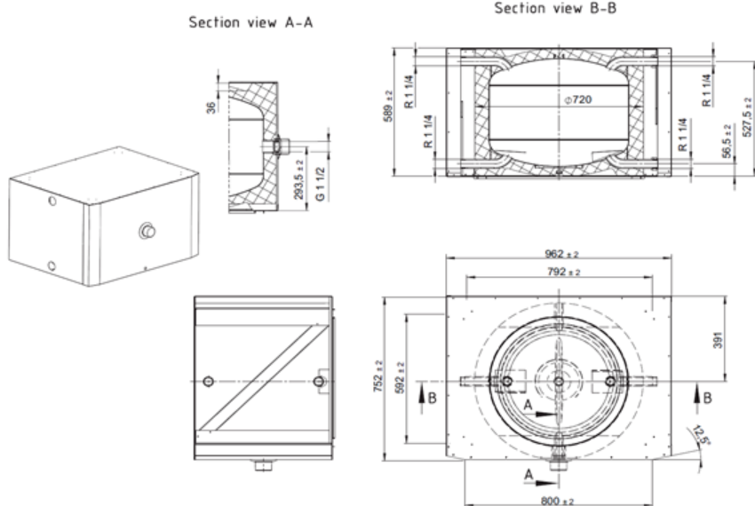
177 Abbildung: Abmessungen des Unterstell-Pufferspeichers PSP 120U für innen aufgestellte Luft/Wasser-Wärmepumpen
