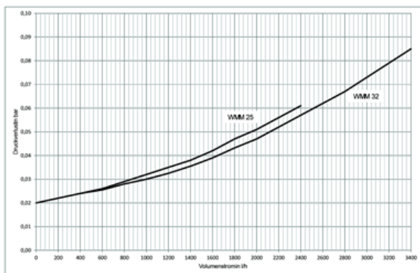
150 Abbildung: Diagramm Druckverlust WMM 25 und WMM 32
