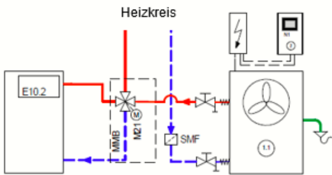
184 Abbildung: 4-Wege-Mischer für den bivalenten Betrieb der Wärmepumpe (Öl- oder Gaskessel)
