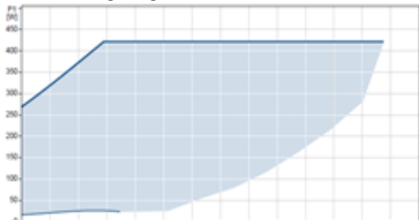
301 Abbildung: Leistungsaufnahme Magna3 40-120F
