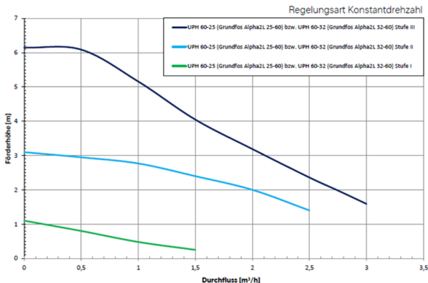
260 Abbildung: Kennlinien UPE 60-25(32)
