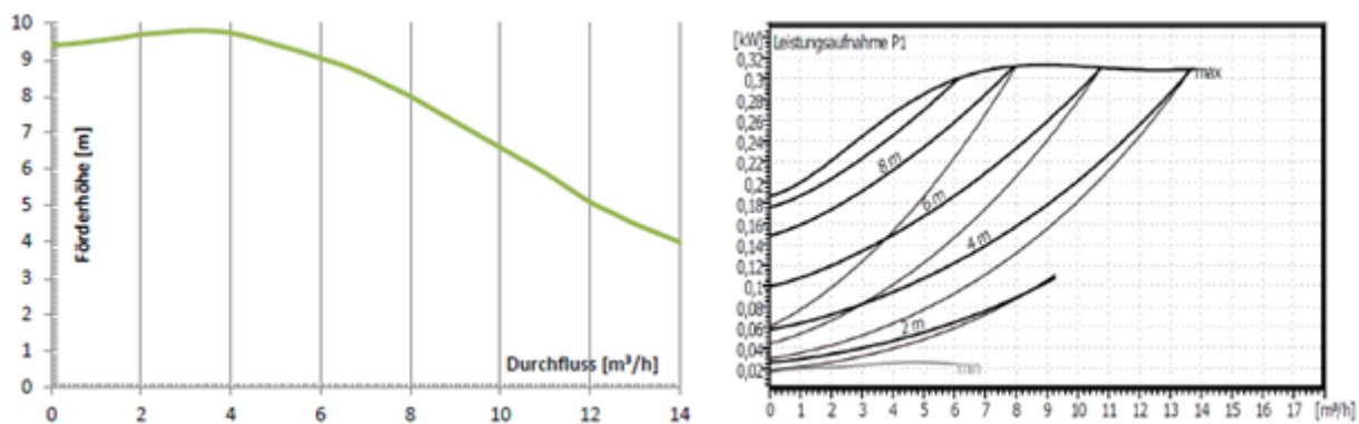
293 Abbildung: Förderhöhe und Leistungsaufnahme Stratos Para 30/1-12
