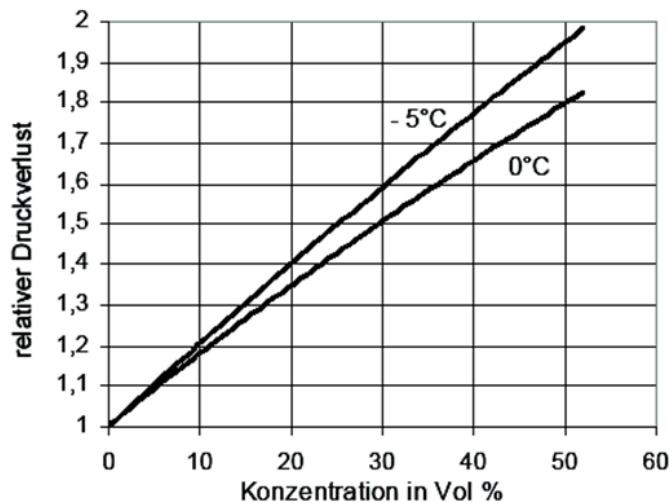
74 Abbildung: Relativer Druckverlust von Monoethylenglykol/Wasser-Gemischen gegenüber Wasser in Abhängigkeit der Konzentration bei 0 °C und -5 °C
