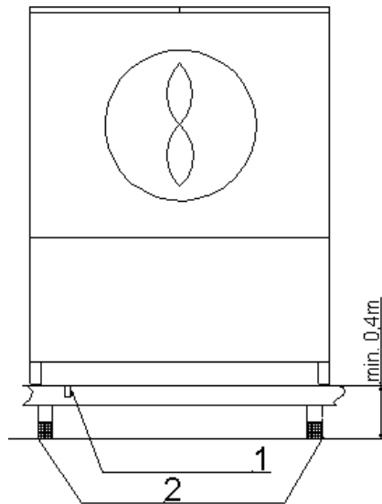
13 Abbildung: Freie Kondensatableitung auf Aufständering (z.B. Gebäudedach)
