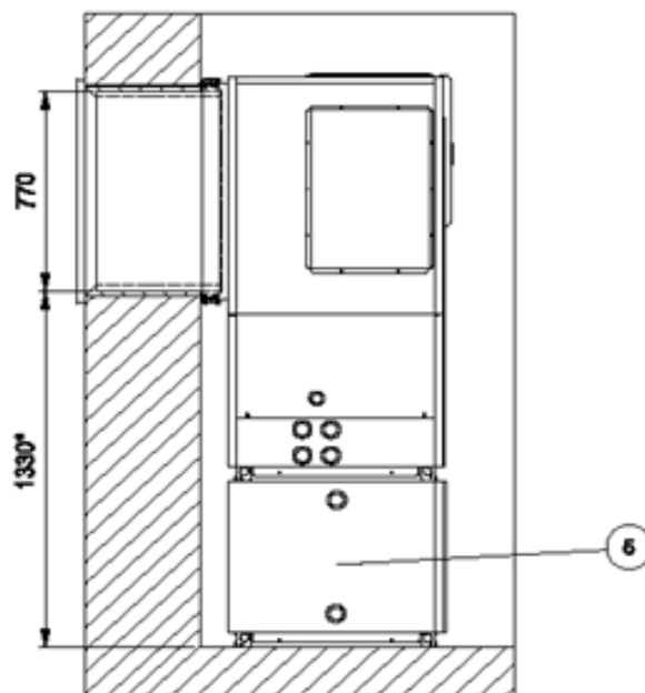
32 Abbildung: Aufstellung mit Unterstellpufferspeicher - Seitenansicht
