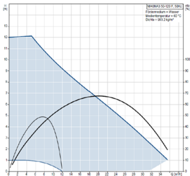
281 Abbildung: Einsatzgrenzen und Kennlinien UPH 120-50F
