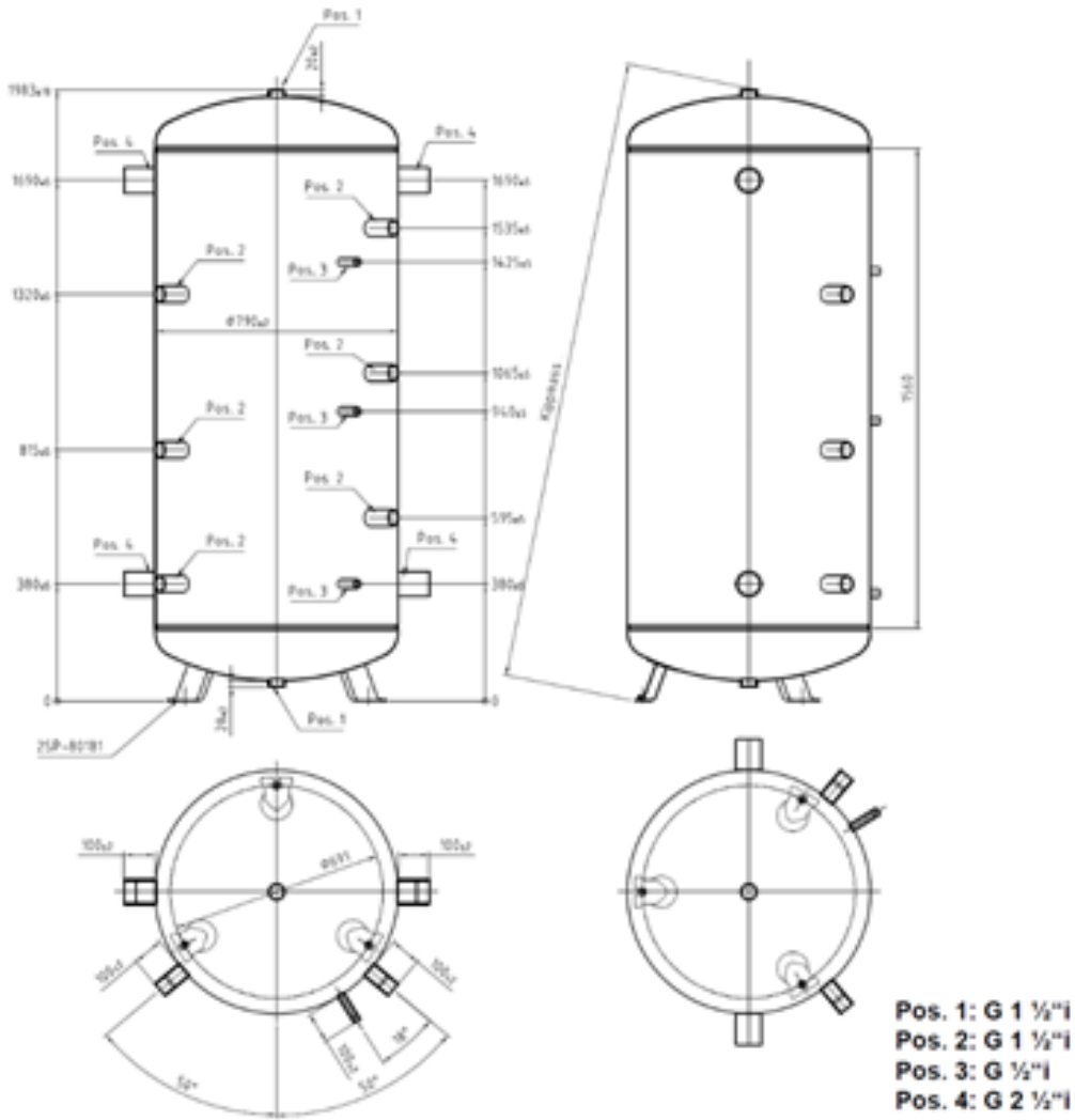
181 Abbildung: Abmessungen Pufferspeicher PSW 1000
