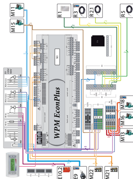
210 Abbildung: Anschlussplan Wärmepumpenmanager WPM EconPlus bei bivalenten Anlagen mit einem Heizkreis und konstant- oder gleitend geregeltem Heizkessel.
