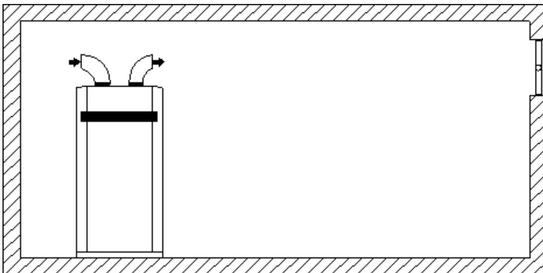
128 Abbildung: Entfeuchten im Umluftbetrieb
