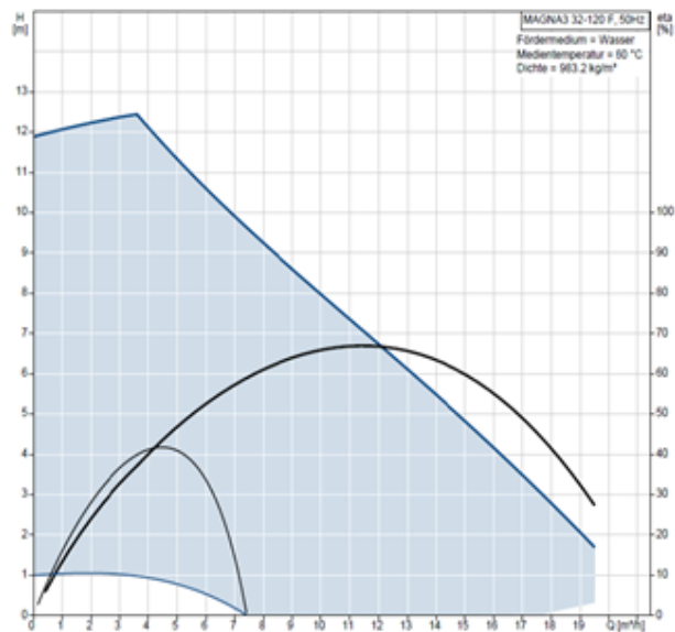
296 Abbildung: Förderhöhe Magna3 32-120F
