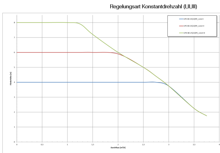
247 Abbildung: Kennlinien UPE 80-25(32) PK
