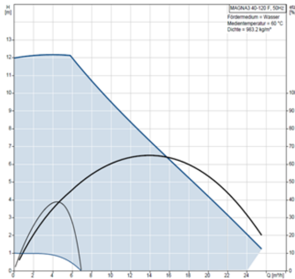
302 Abbildung: Förderhöhe Magna3 40-120F
