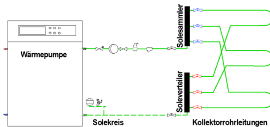
80 Abbildung: Wärmepumpenkreislauf Wärmequellenseite
