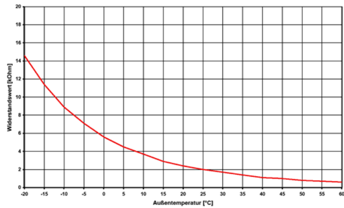
132 Abbildung: Fühlerkennlinie NTC-10 zum Anschluss an den Heizungsregler
