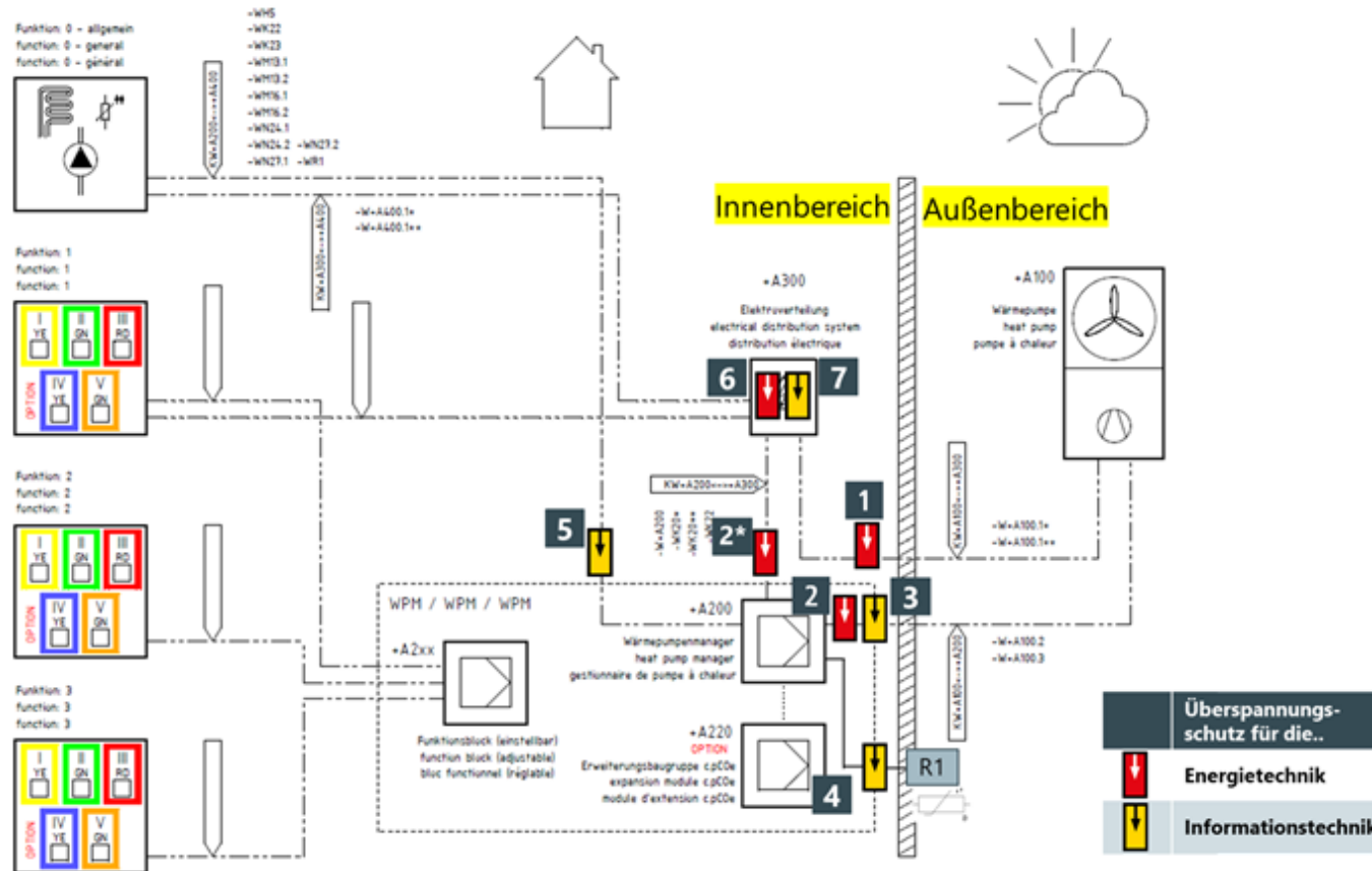
9 Abbildung: Blitz- und Überspannungsschutzkonzept am Beispiel System M / M Flex
