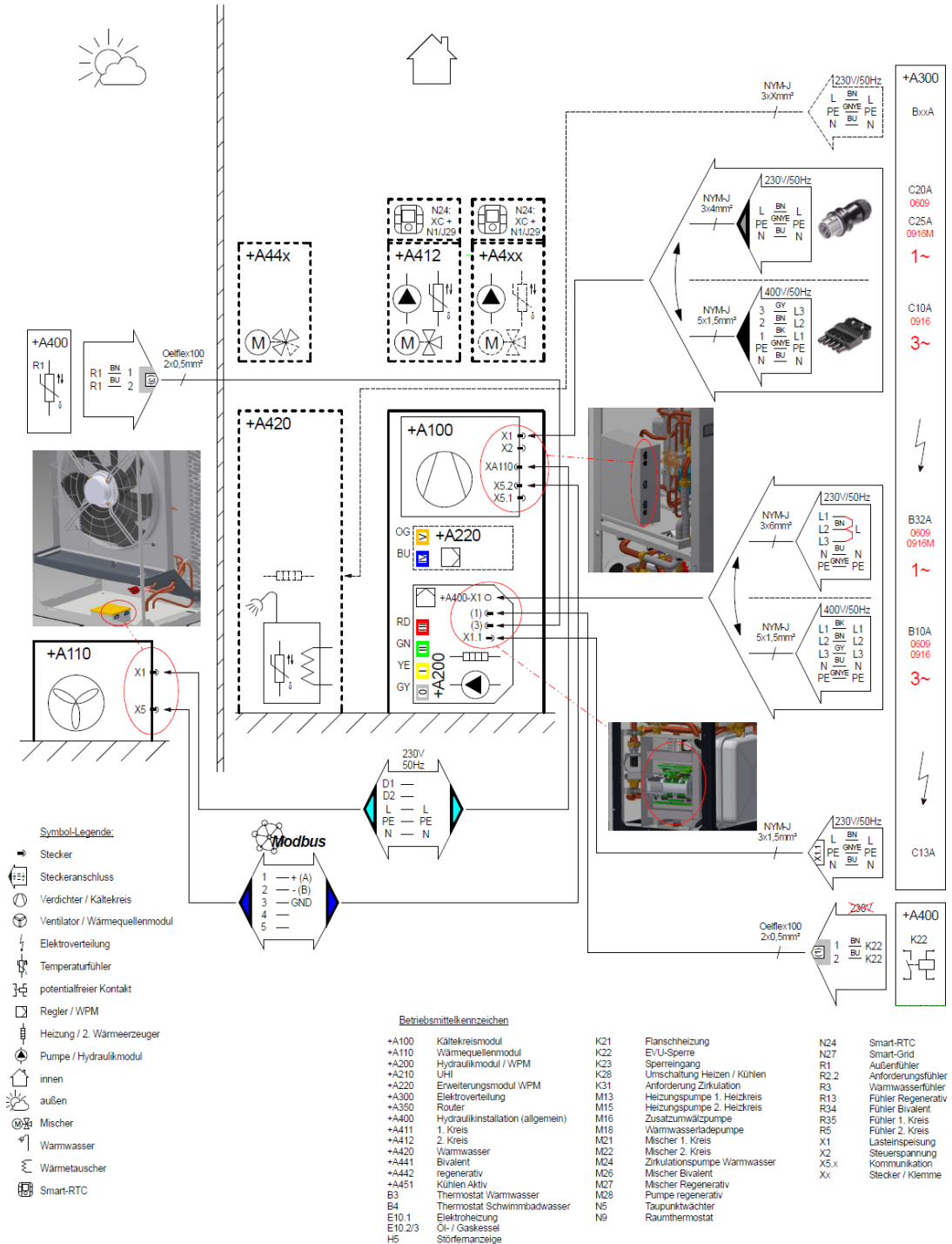
71 Abbildung: Anschlussplan M Flex 0609 (230V), 0916(M) (230 / 400V)
