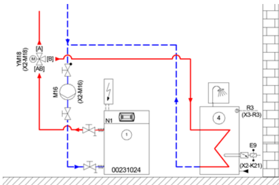
189 Abbildung: Warmwasserbereitung über 3-Wege Ventil
