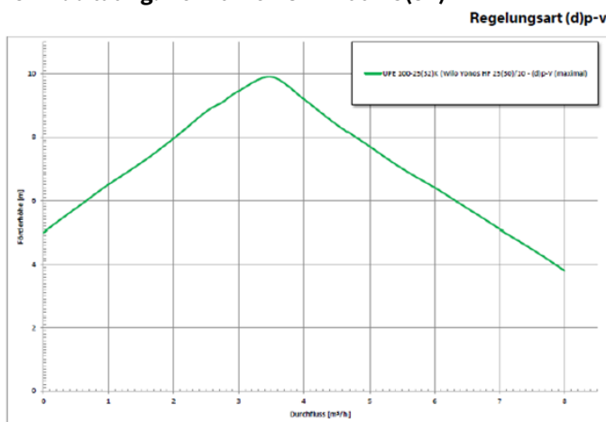
253 Abbildung: Kennlinien UPE 100-25(32)K
