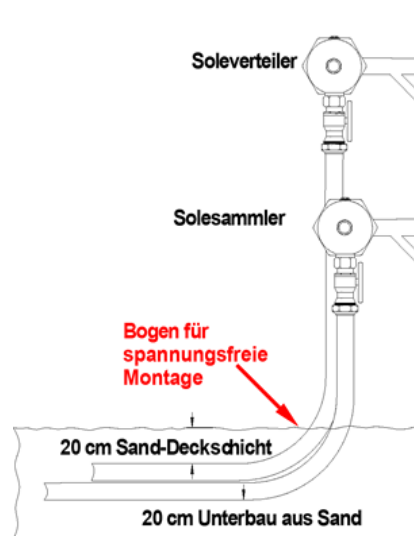
78 Abbildung: Montage der Rohrleitungen am Soleverteiler
