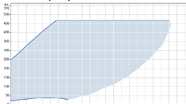
307 Abbildung: Leistungsaufnahme Magna3 65-80F
