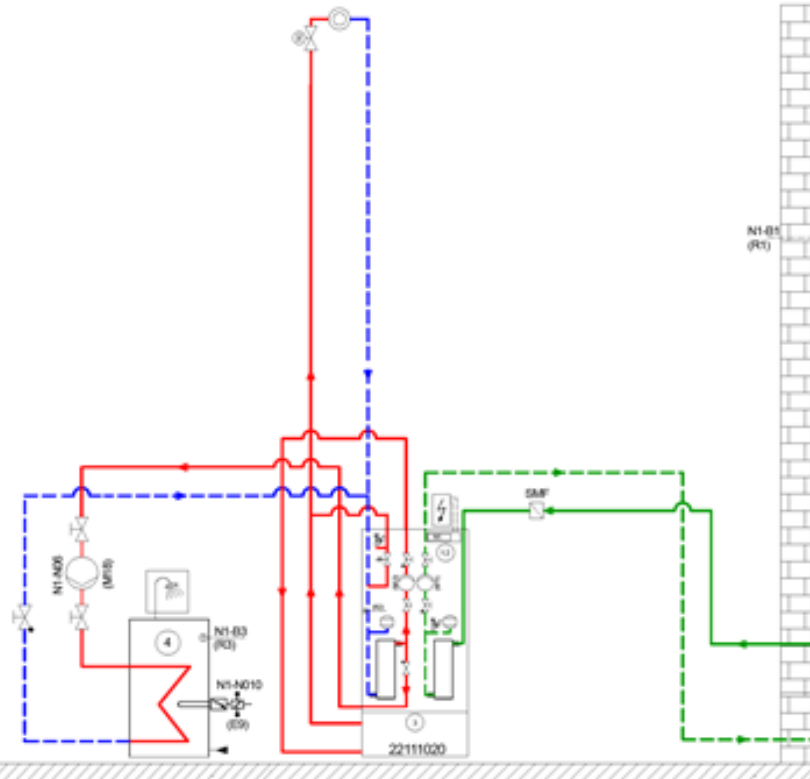
197 Abbildung: Einbindungsschema für den monovalenten Wärmepumpenbetrieb mit einem Heizkreis und Unterstellpuffer
