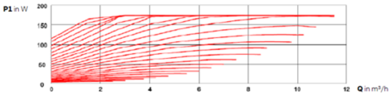
291 Abbildung: Förderhöhe und Leistungsaufnahme MagnaGeo 32-100VDC
