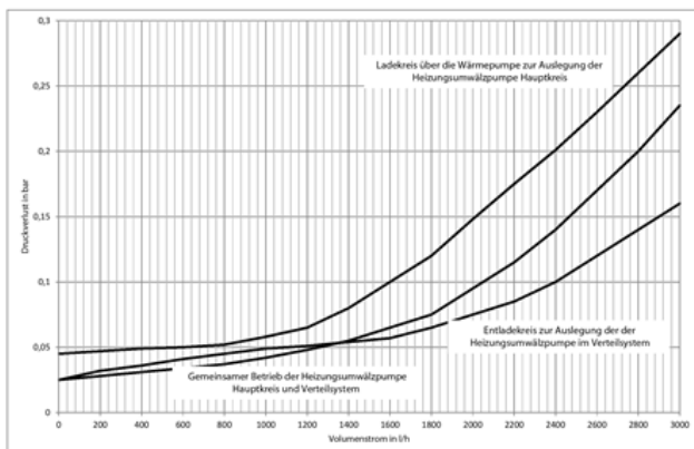
161 Abbildung: Volumenstrom-Druckverlust-Diagramm DDV 25 / DDV 32
