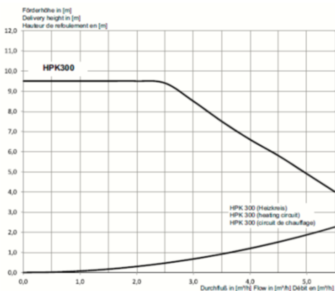
172 Abbildung: Pumpen- / Gerätekenlinie Verbraucherkreis HPK 300
