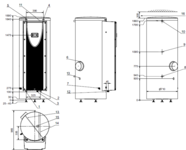
169 Abbildung: Abmessungen HWK 332 (Econ5S)
