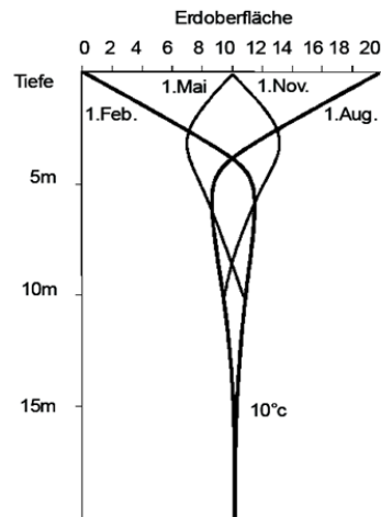
82 Abbildung: Darstellung des Temperaturverlaufs in unterschiedlichen Tiefen des Erdreichs und in Abhängigkeit eines jahreszeitlichen, mittleren Temperaturwertes an der Erdoberfläche
