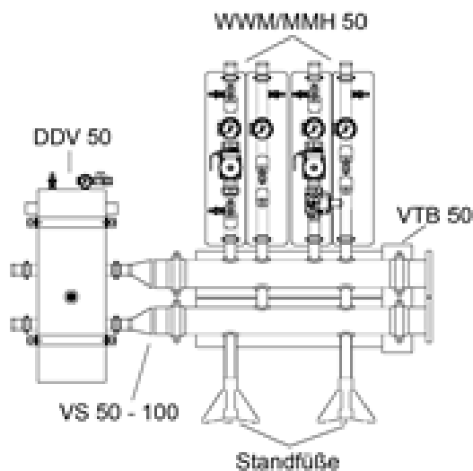
164 Abbildung: Einbindung des doppelt differenzdrucklosen Verteilers DDV 50 für Heizbetrieb und Warmwasserbereitung
