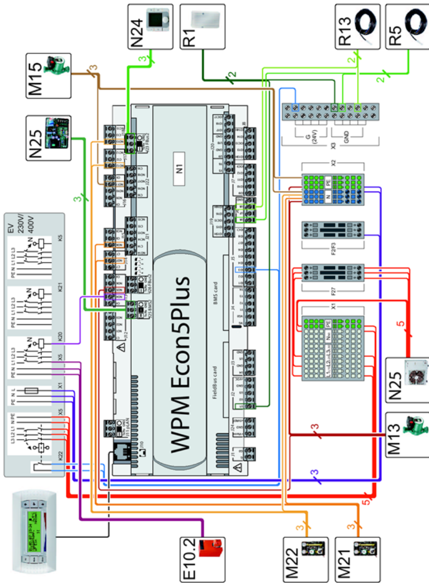
328 Abbildung: Anschlussplan des Wärmepumpenmanagers WPM Econ5Plus für die Wärmepumpen LAW 9IMR und LAW 14ITR
