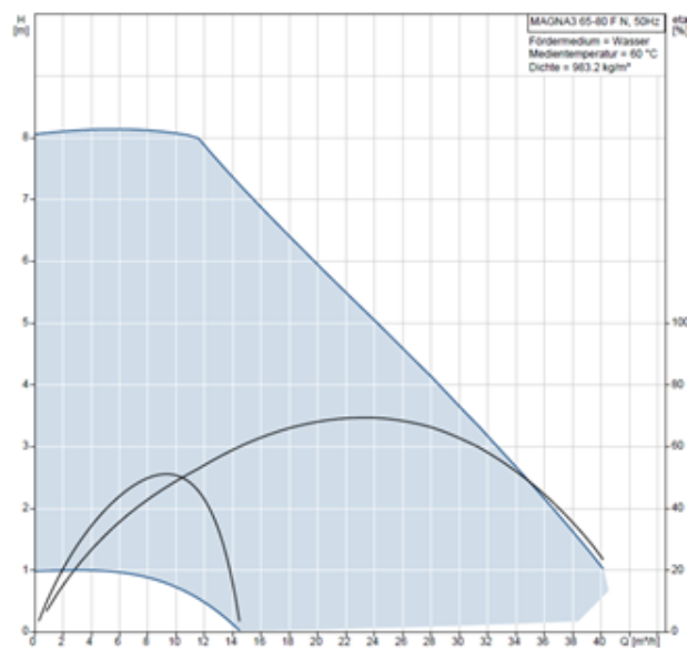
308 Abbildung: Förderhöhe Magna3 65-80F
