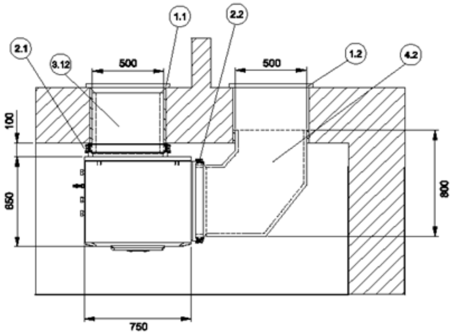
39 Abbildung: Draufsicht - LIK 8TES (Wand-Aufstellung - Luftkanal Ausblasseite)
