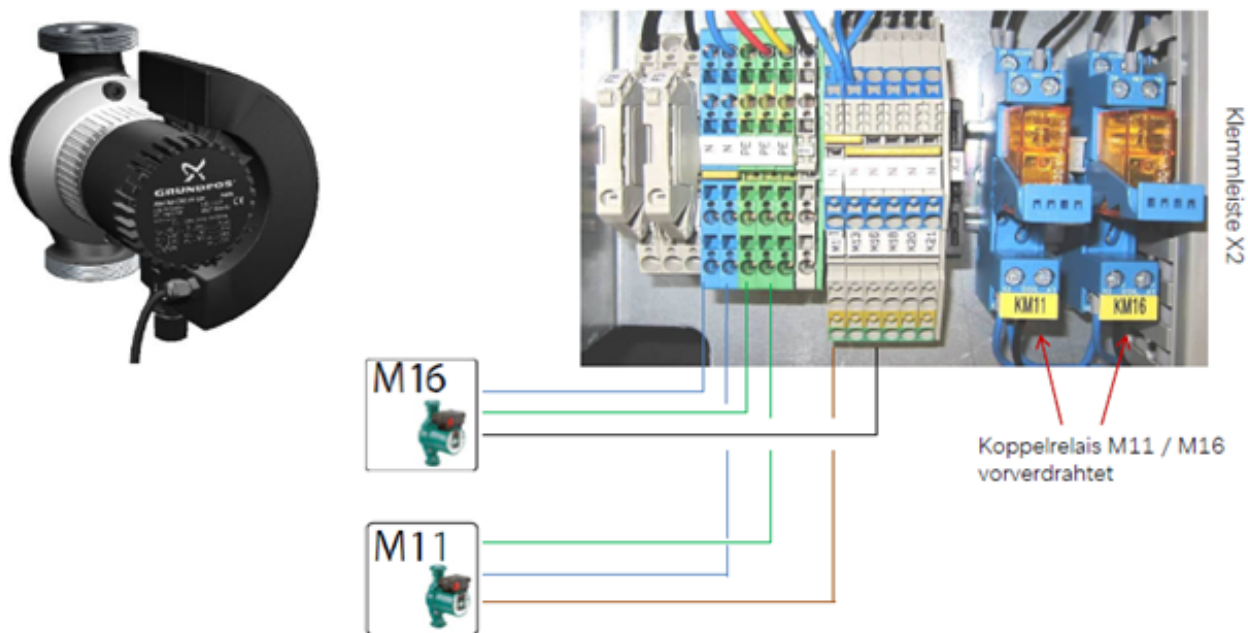
318 Abbildung: Elektrischer Anschluss 230V Erzeuger- und Wärmequellen- (Sole-)Pumpe
