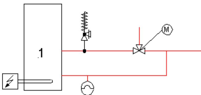
173 Abbildung: Heizsystem mit konstant geregelttem Pufferspeicher
