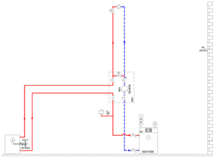
202 Abbildung: Einbindungsschema für den monoenergetischen Wärmepumpenbetrieb mit einem Heizkreis und Reihen-Pufferspeicher
