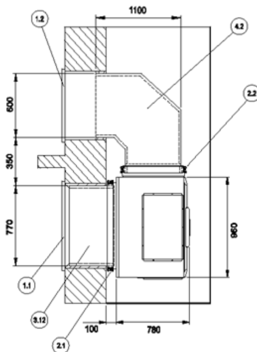
34 Abbildung: Draufsicht - LI 12TU und LI 16I-TUR (Wand-Aufstellung - Luftkanal Ausblasseite)
