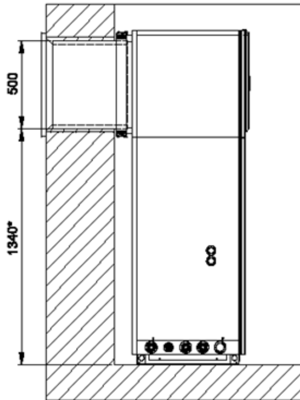
36 Abbildung: Seitenansicht - LIK 8TES (Eck-Aufstellung)
