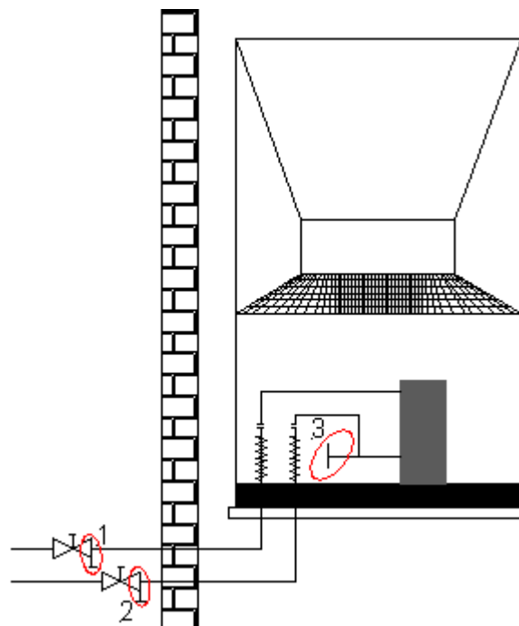
14 Abbildung: Entleerungsstellen bei Luft/Wasser-Wärmepumpen
