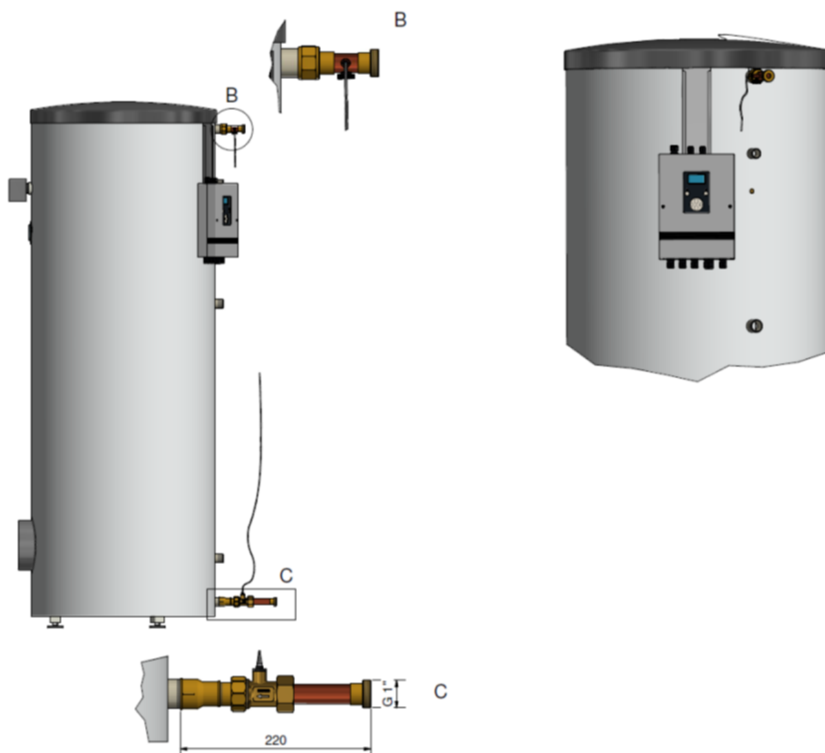
111 Abbildung: Hydraulischer Aufbau DFM 1988-1
