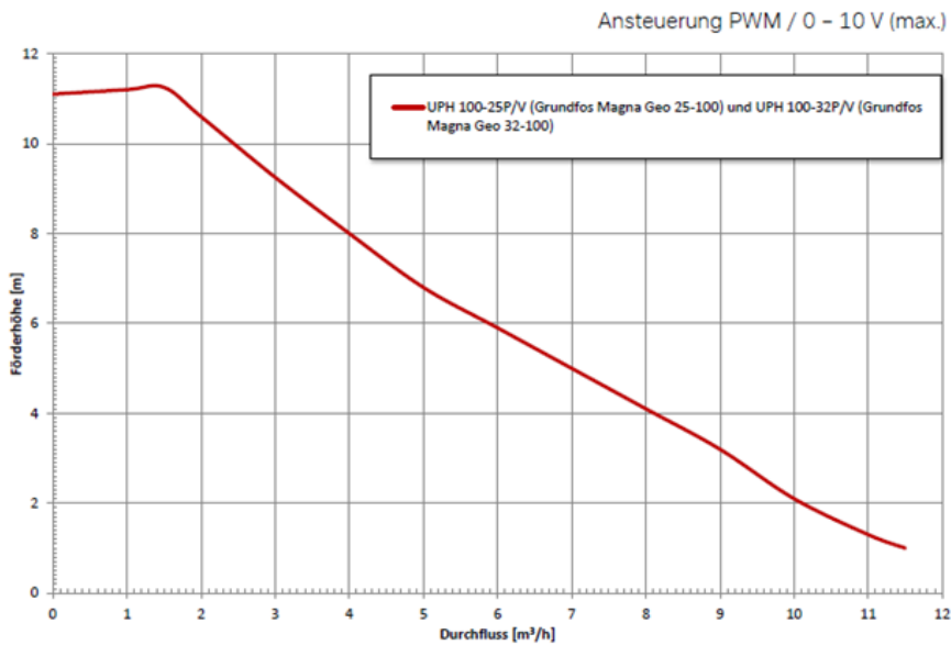
272 Abbildung: Kennlinien UPH 100-25(32) P und UPH 100-25(32) V
