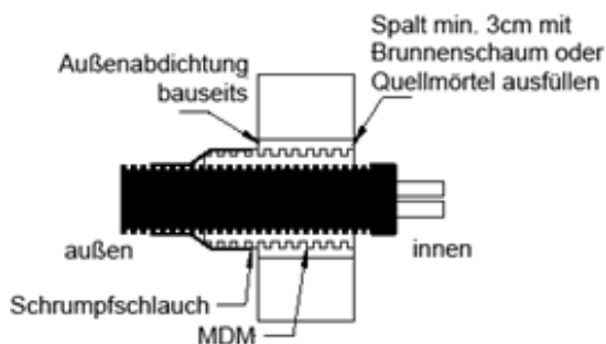
22 Abbildung: Skizze Mauerdurchführung nicht drückendes Wasser
