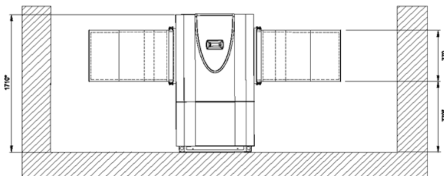
54 Abbildung: Frontansicht - LI 1422C und LI 1826C (Wand-Aufstellung mit Luftkanal auf der Ansaug- und Ausblasseite)
