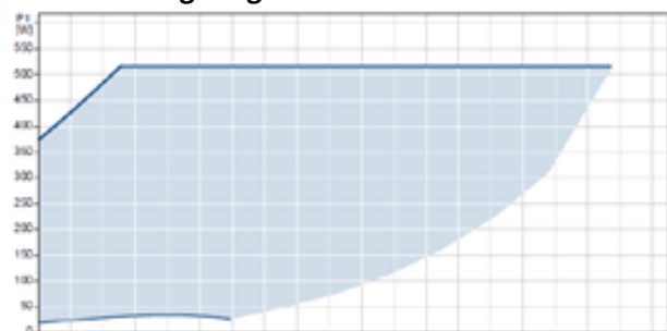
304 Abbildung: Leistungsaufnahme Magna3 50-120F
