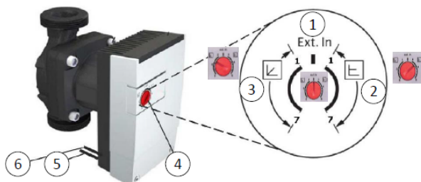
273 Abbildung: Einstellungsmöglichkeiten UPH 120-32 PK
