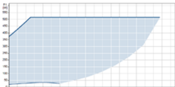
280 Abbildung: Einsatzgrenzen und Kennlinien UPH 120-50F
