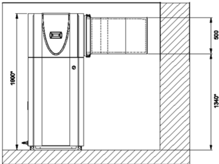
40 Abbildung: Frontansicht - LIK 8TES (Wand-Aufstellung - Luftkanal Ausblasseite) LI 12TU und LI 16I-TUR - Eck-Aufstellung
