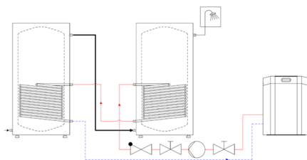
103 Abbildung: Reihenschaltung von Warmwasserspeichern
