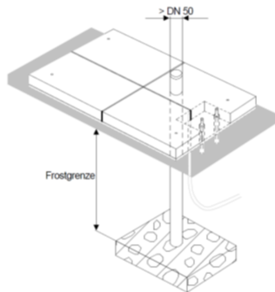
16 Abbildung: Skizze Fundament mit Gehwegplatten
