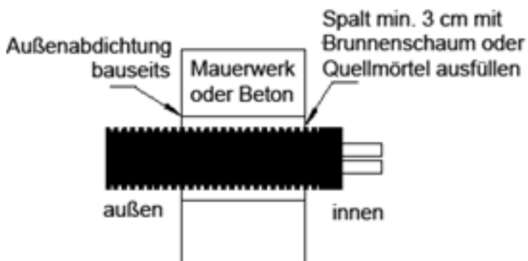
21 Abbildung: Skizze direkte Mauerdurchführung
