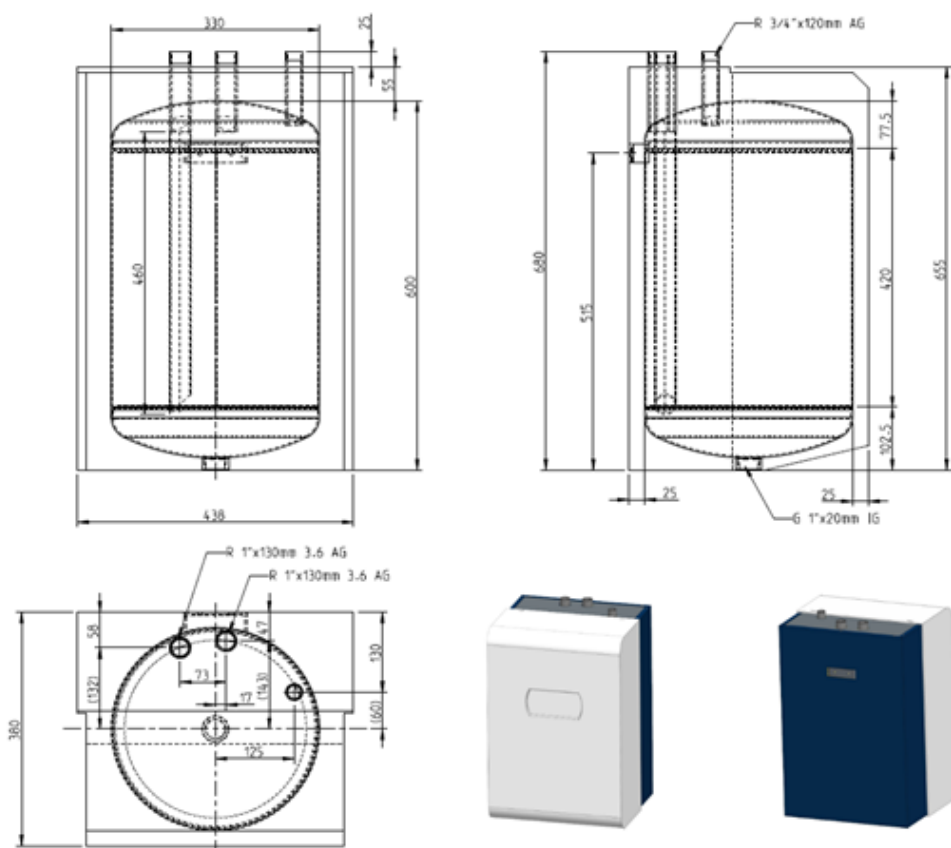
174 Abbildung: Abmessungen des wandhängenden Pufferspeichers PSP 50E
