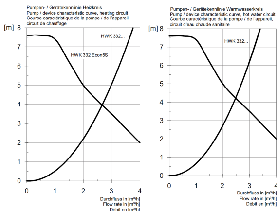
168 Abbildung: Pumpen-, Gerätekenlinie - Heizkreis - Warmwasserkreis HWK 332 Econ5S
