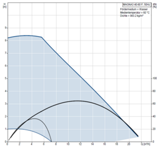
299 Abbildung: Förderhöhe Magna3 40-80F
