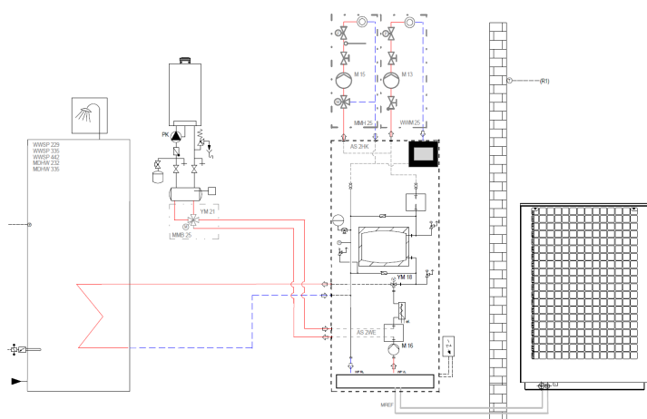
229 Abbildung: Einbindungsschema mit integriertem Pufferspeicher, Erzeuger- und Verbraucherkreisen, Warmwasserspeicher und bivalentem Wärmeerzeuger
