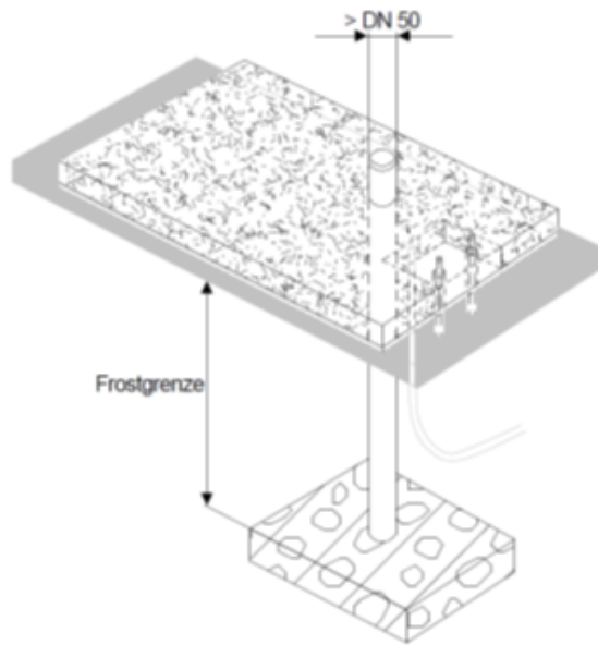
15 Abbildung: Skizze Betonfundament
