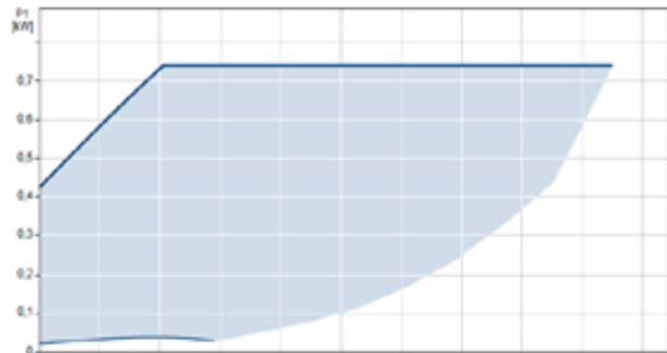
313 Abbildung: Leistungsaufnahme Magna3 65-120F
