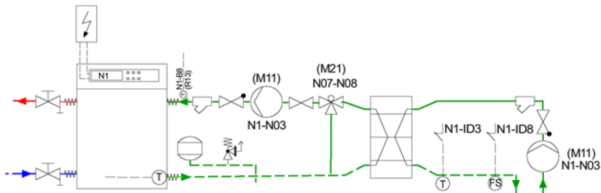
87 Abbildung: Wärmepumpe mit thermostatisch geregelttem 3-Wege-Ventil im Solekreislauf M21 (bauseits zu stellen)
