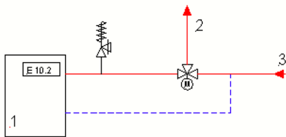
186 Abbildung: Schaltbild für gleitend geregelten Heizkesselbetrieb
