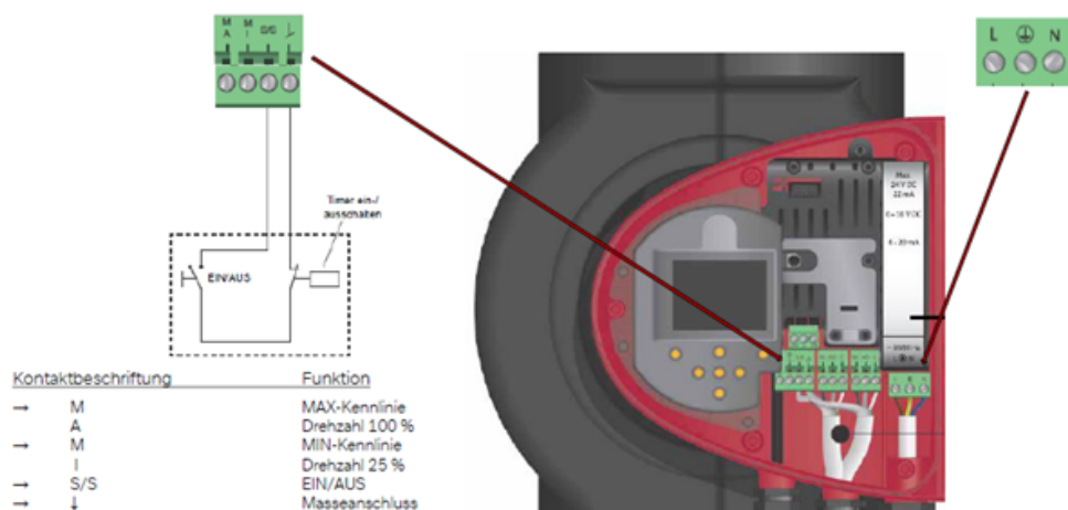
323 Abbildung: Elektrischer Anschluss Digitaleingang Magna3-Baureihe
