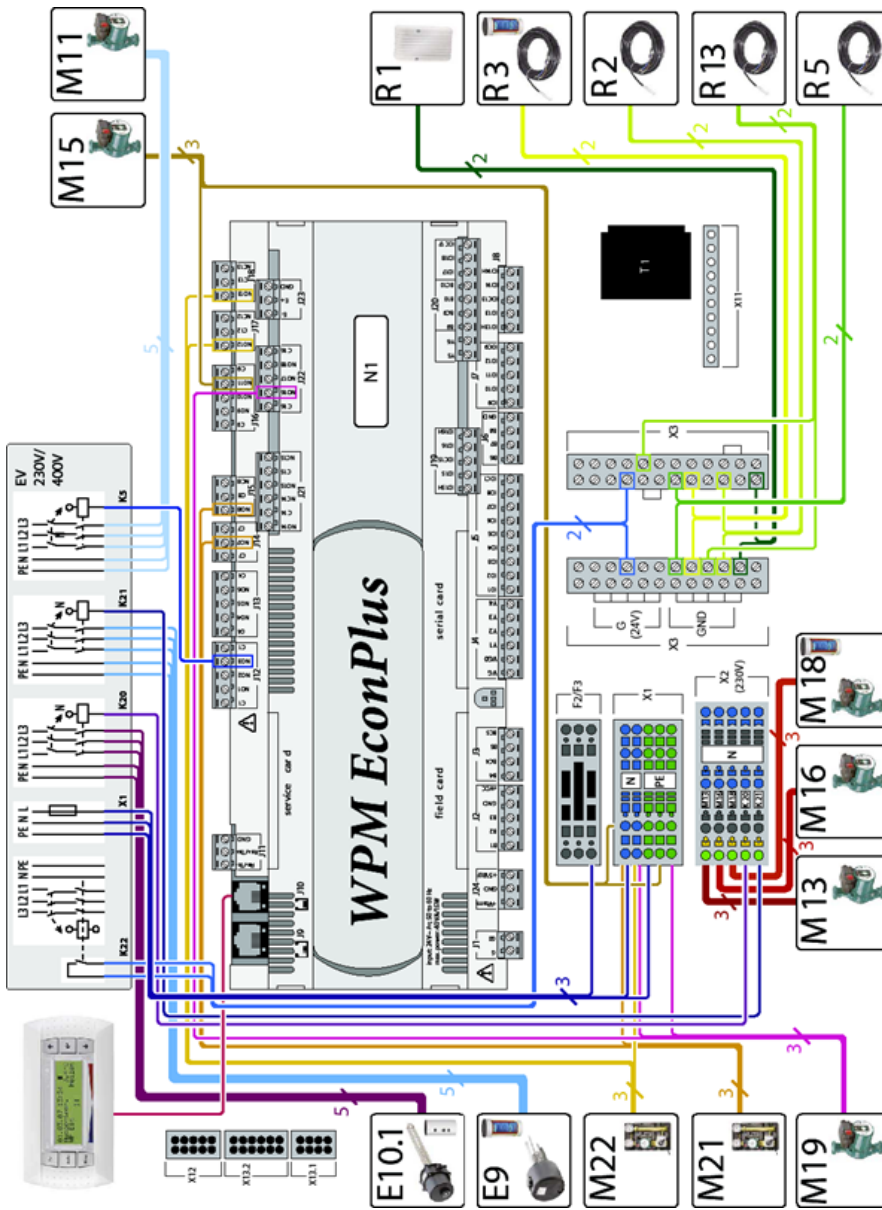
327 Abbildung: Anschlussplan des wandmontierten Wärmepumpenmanagers WPM EconPlus
