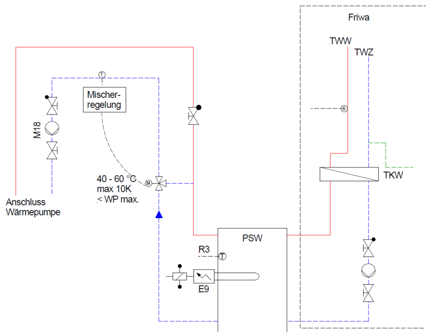
118 Abbildung: Hydraulische Einbindung Frischwasserstation mit Rücklaufanhebung
