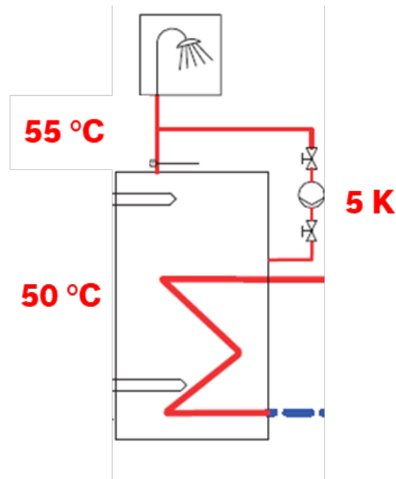
109 Skizze: Zulässige Temperaturen bei Anlagen mit hohem Wasseraustausch nach DIN 1988-200
