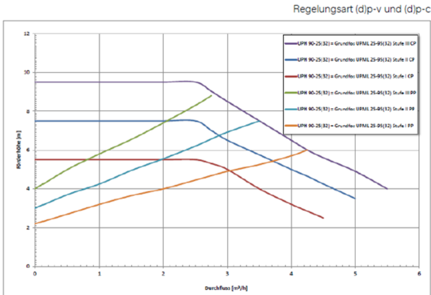
268 Abbildung: Kennlinien UPH 90-25(32)
