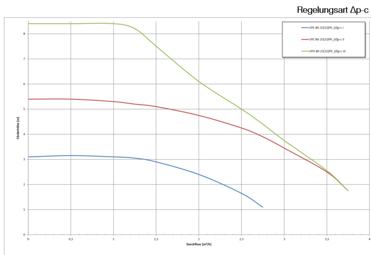
248 Abbildung: Kennlinien UPE 80-25(32) PK
