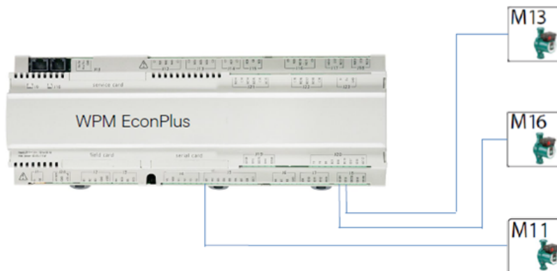
285 Abbildung: Elektrische Verdrahtung Steuersignal 0 - 10V am WPM EconPlus
