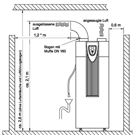
125 Abbildung: Aufstellungsbedingungen für freies Ansaugen und Ausblasen der Prozessluft.
