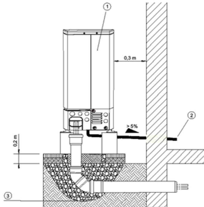
55 Abbildung: Kondensatablauf LIA-Wärmepumpen
