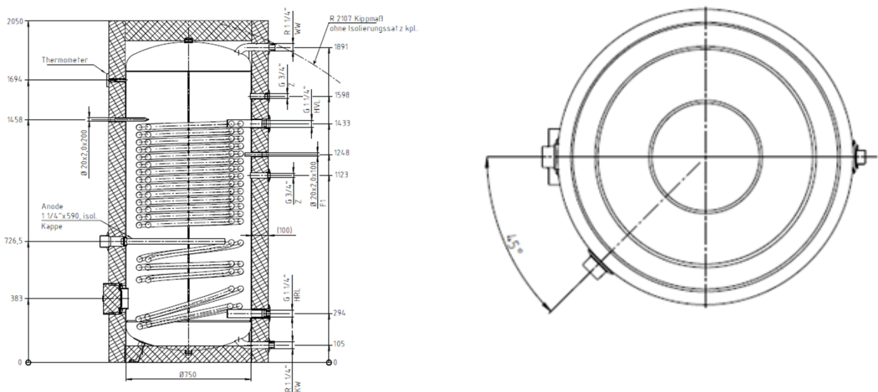
116 Abbildung: Zeichnung WWSP 770
