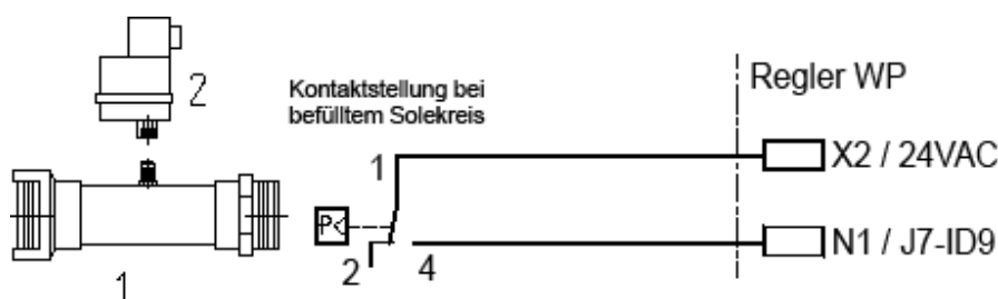
85 Abbildung: Niederdruckpressostat Sole (Aufbau und Verschaltung)
