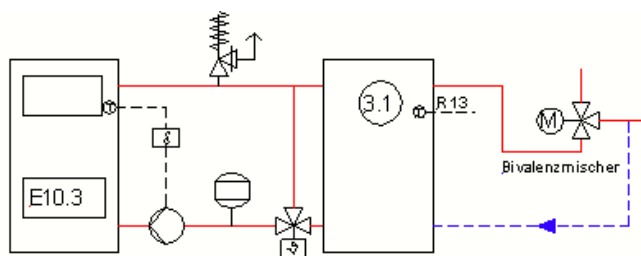
187 Abbildung: Schaltbeispiel für den Heizbetrieb mit Festbrennstoffkessel
