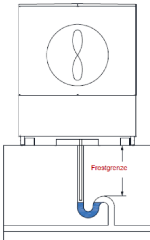
12 Abbildung: Kondensatablauf in Kanal (Darstellung mit Siphon)
