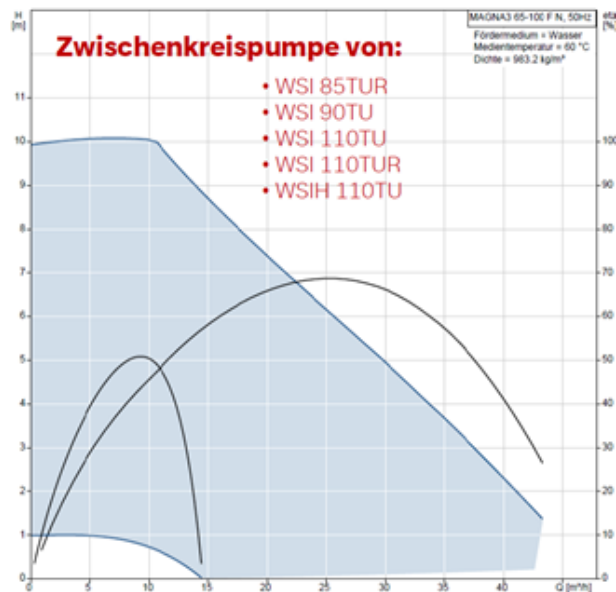
311 Abbildung: Förderhöhe Magna3 65-100F
