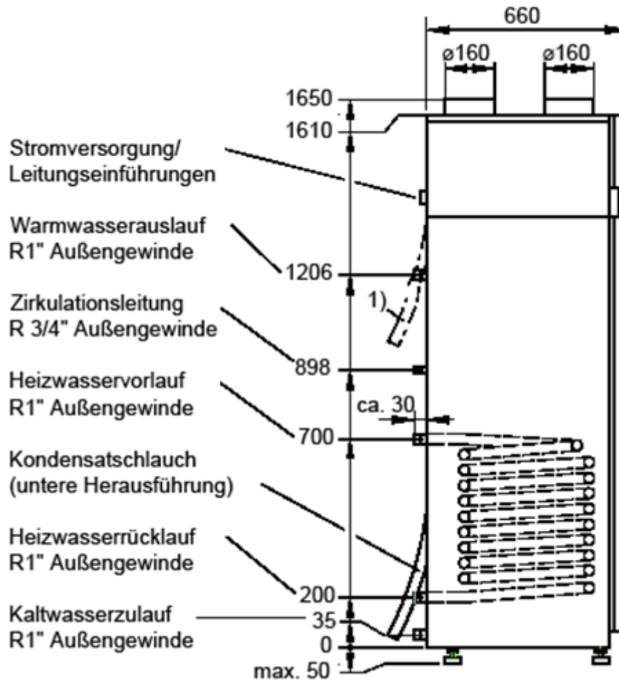
123 Abbildung: Anschlüsse und Abmessungen der Warmwasser-Wärmepumpe mit innen liegendem Zusatz-Wärmeübertrager 1) alternative Kondensatführung
