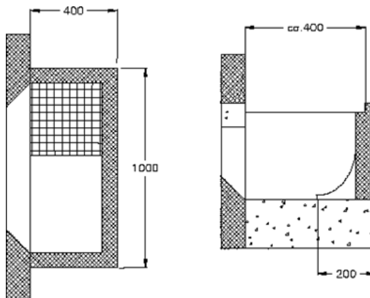
27 Abbildung: Beispiel: Abmessungen für Standard-Lichtschächte
