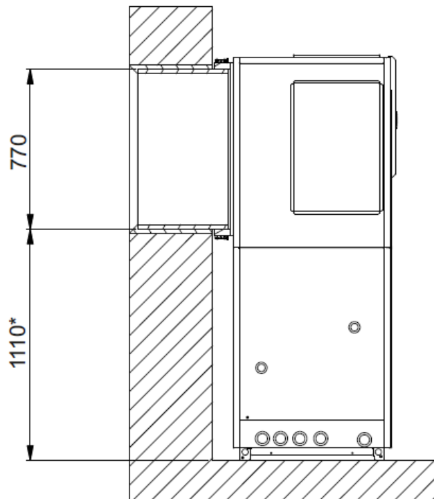
46 Abbildung: Seitenansicht - LIK 12TU
