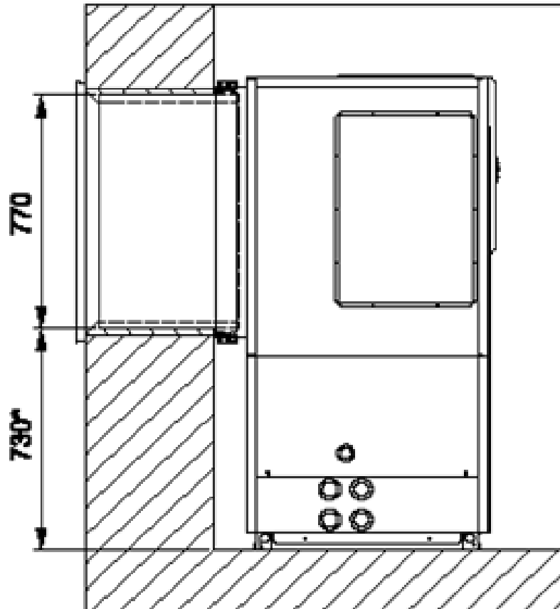
41 Abbildung: Seitenansicht - LI 12TU und LI 16I-TUR
