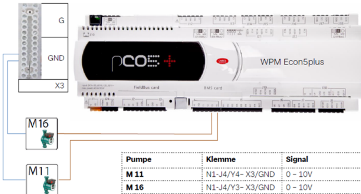
319 Abbildung: Elektrischer Anschluss Steuersignal 0 - 10V Erzeuger- und Wärmequellen- (Sole-)Pumpe
