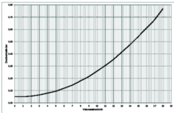
149 Abbildung: Diagramm Druckverlust MMH 50
