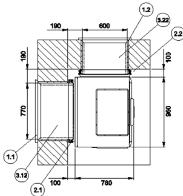
42 Abbildung: Draufsicht - LI 12TU und LI 16I-TUR (Eck-Aufstellung)
