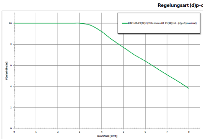
252 Abbildung: Kennlinien UPE 100-25(32)K
