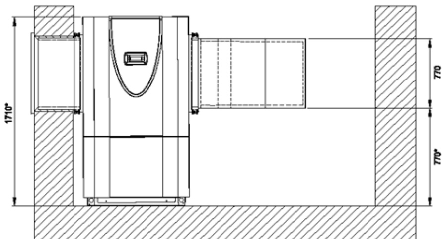
52 Abbildung: Frontsicht - LI 1422C und LI 1826C (Wand-Aufstellung mit Luftkanal auf der Ausblasseite) LI 1422C und LI 1826C - Wand-Aufstellung mit Luftkanälen auf der Ansaug- und Ausblasseite
