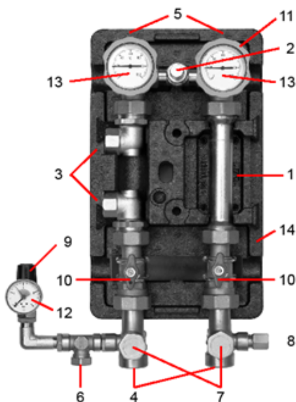
154 Abbildung: Aufbau Kompaktverteiler KPV 25
