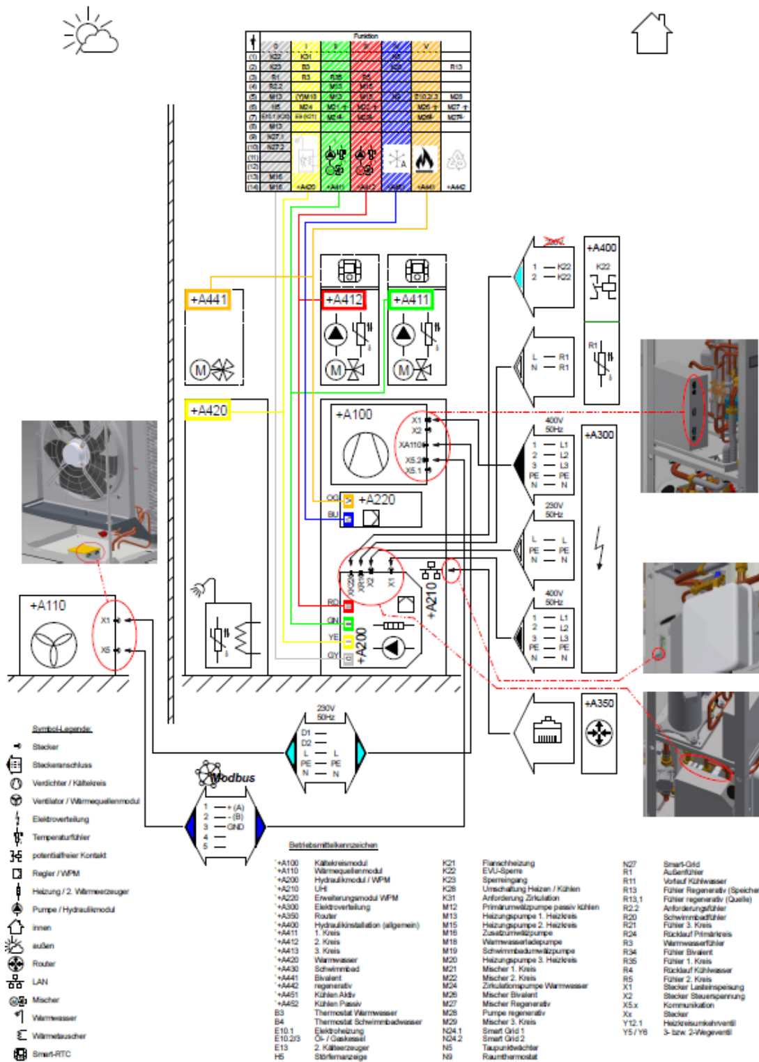
70 Abbildung: Anschlussplan System M Comfort (230 / 400V)
