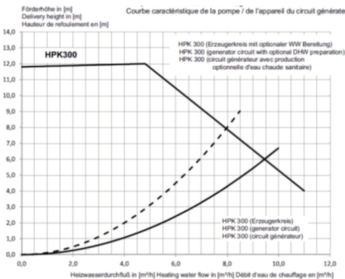
171 Abbildung: Pumpen- / Gerätekenlinie Erzeugerkreis HPK 300
