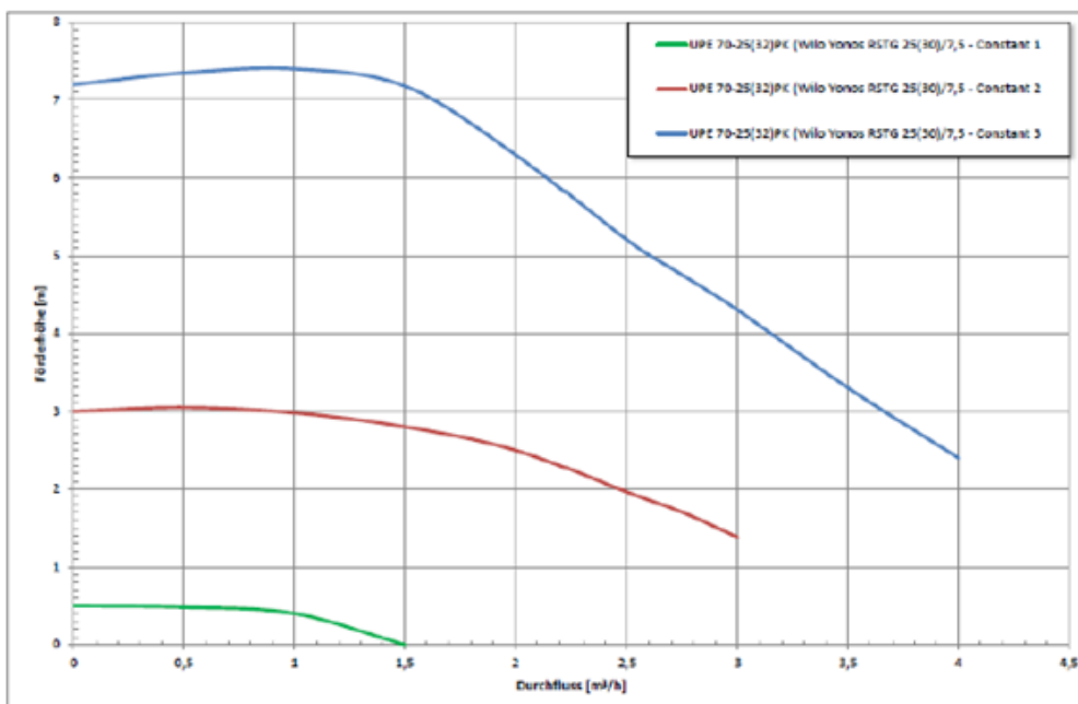
246 Abbildung: Kennlinien UPE 70-25(32)PK
