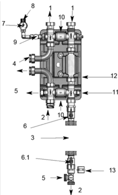
159 Abbildung: Doppelt differenzdrucklosen Verteiler DDV zum Anschluss eines gemischten Heizkreises, externer Heizungsunterstützung und optionaler Warmwasserbereitung.
