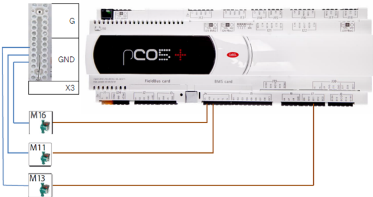
283 Abbildung: Elektrische Verdrahtung des Steuersignals am Wärmepumpenmanager WPM Econ5plus
