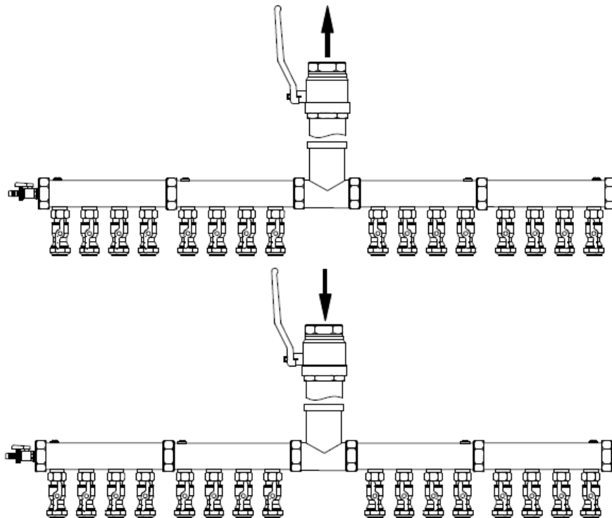
77 Abbildung: Montage Soleverteiler für max. 16 (2 x 8) Kreise
