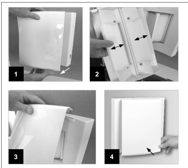
Abb. 7.1 Filterwechsel
