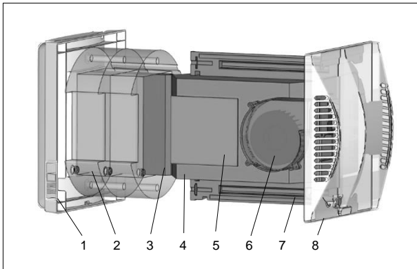
Abb. 2.3 Prinzipieller Geräteaufbau
