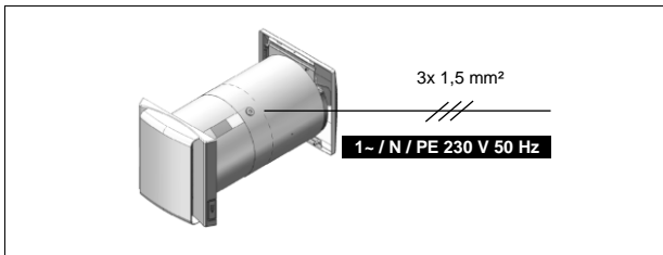
Abb. 4.13 Spannungsversorgung Lüftungsgerät
