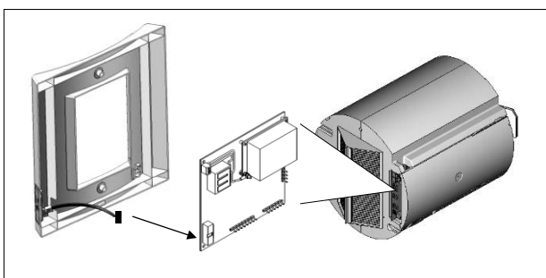
Abb. 4.14 Anschluss Bedieneinheit
